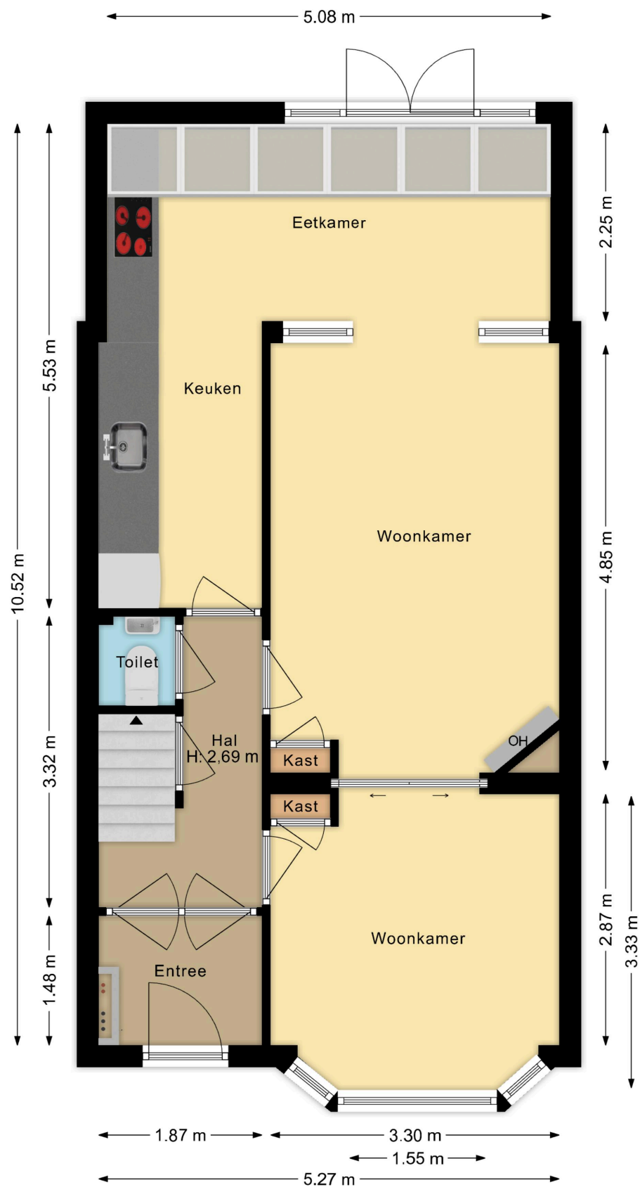
Batavierenplantsoen 48, Haarlem Begane grond
