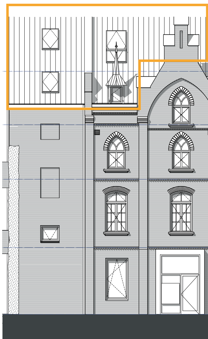
Voorgevel
