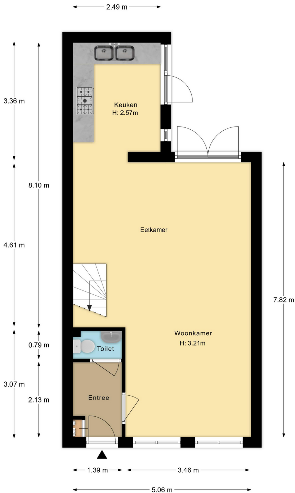
Teylershofjestraat 8 Haarlem Begane Grond
