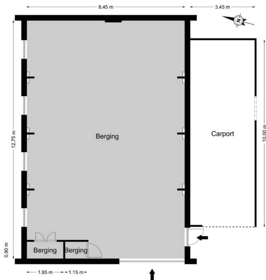
Bijgebouw - 2D
