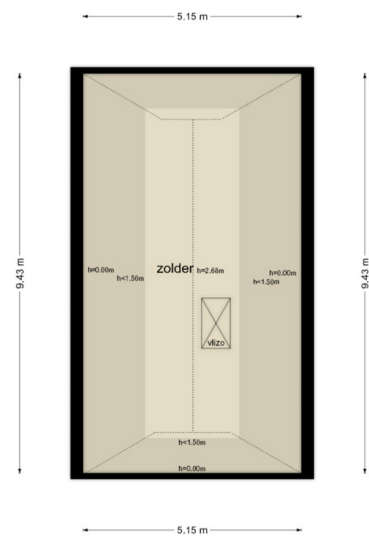
Vliering
