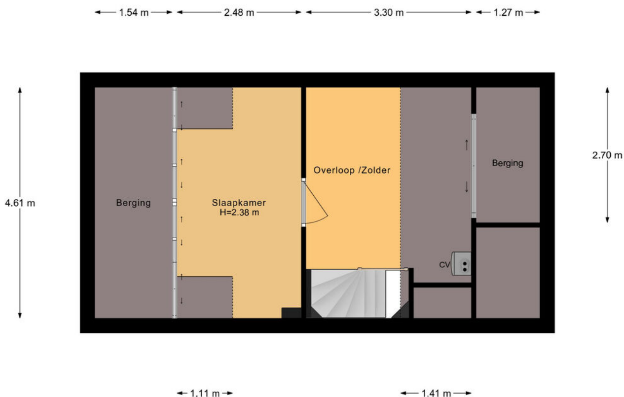
2e Verdieping
