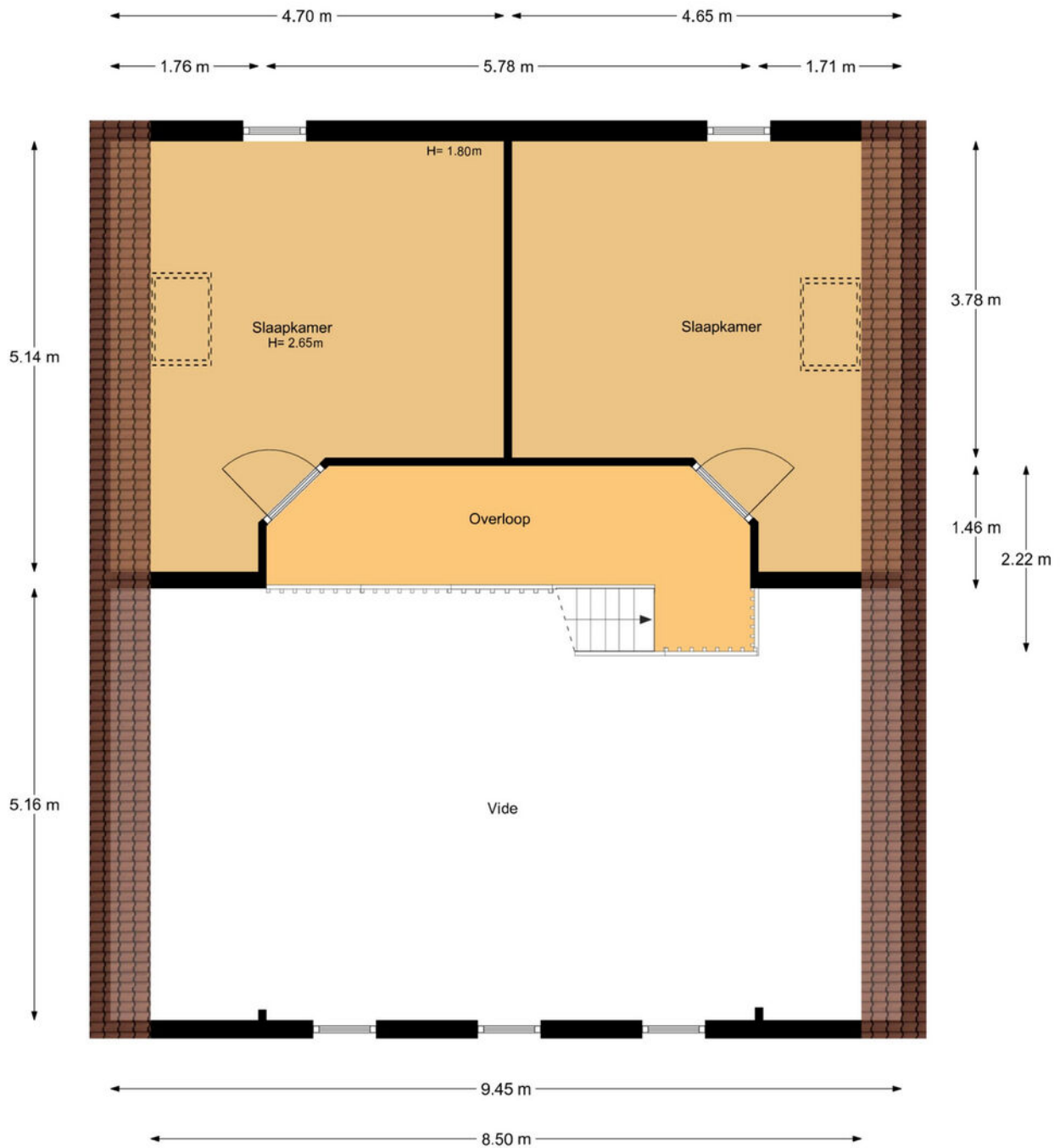
Bijgebouw - 1e verdieping
