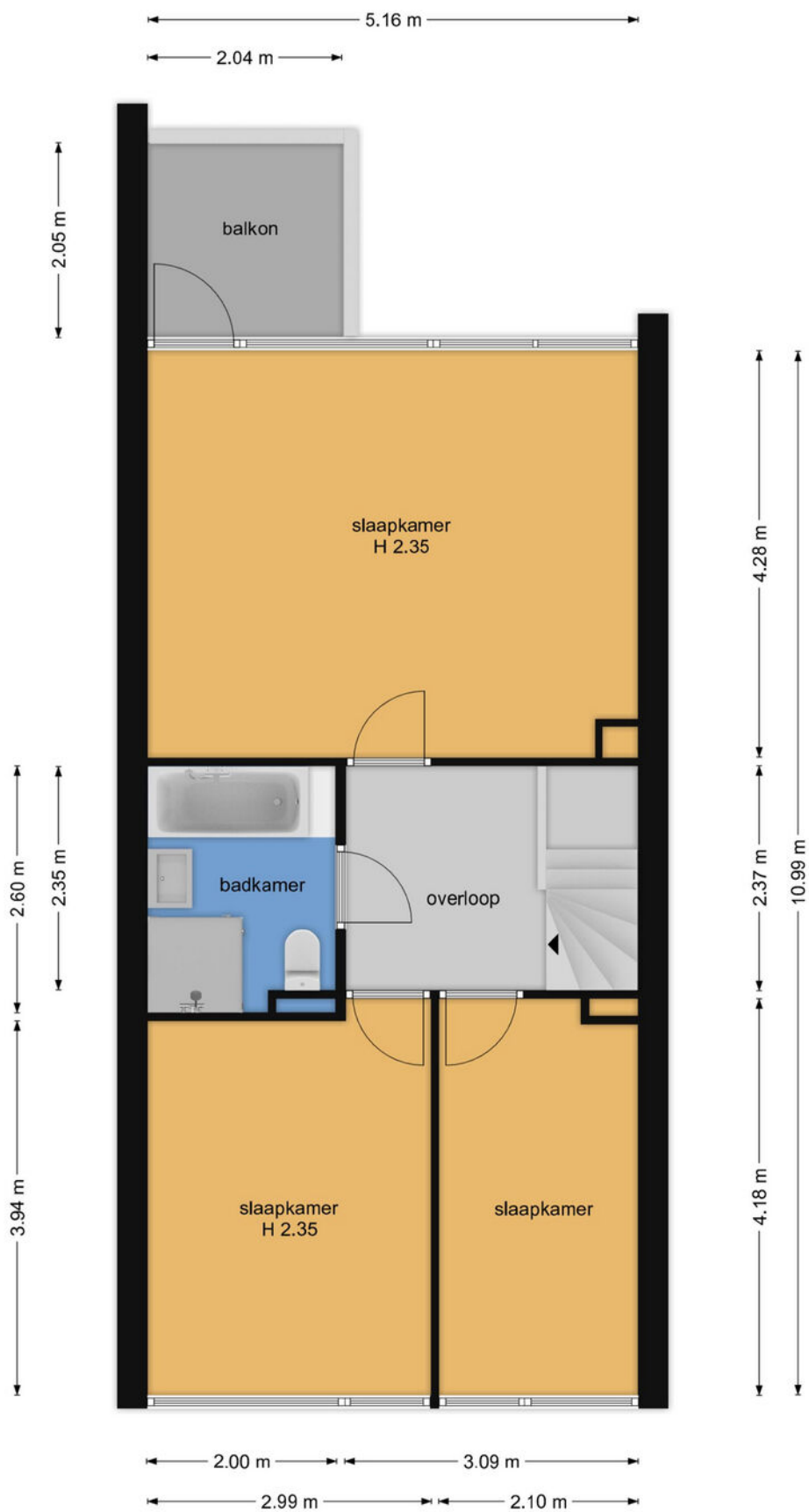
1e verdieping
