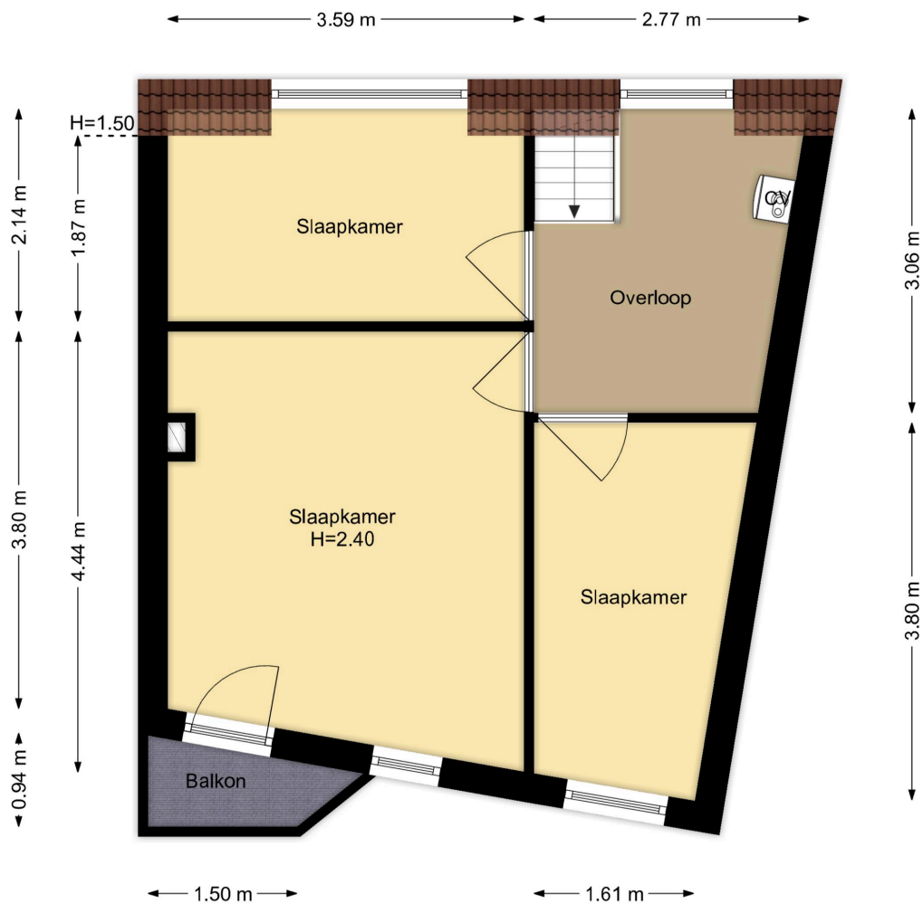
2e Verdieping Benkoelenstraat 27, Haarlem R.M. Vastgoedpresentatie| Aan deze plattegrond kunnen geen rechten worden ontleend
