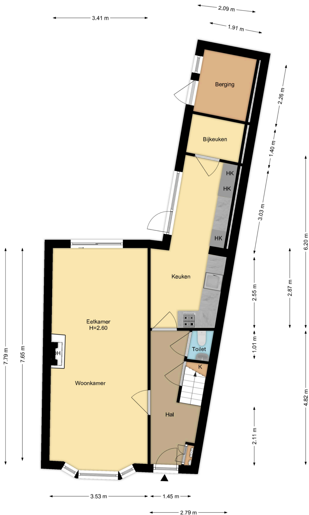
Begane Grond Benkoelenstraat 27, Haarlem R.M. Vastgoedpresentatie| Aan deze plattegrond kunnen geen rechten worden ontleend
