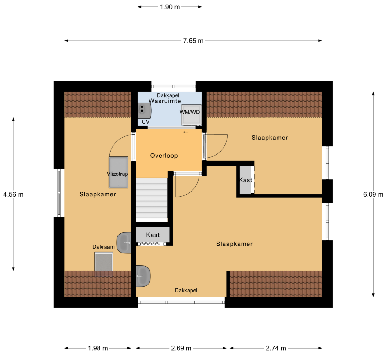
1e Verdieping
