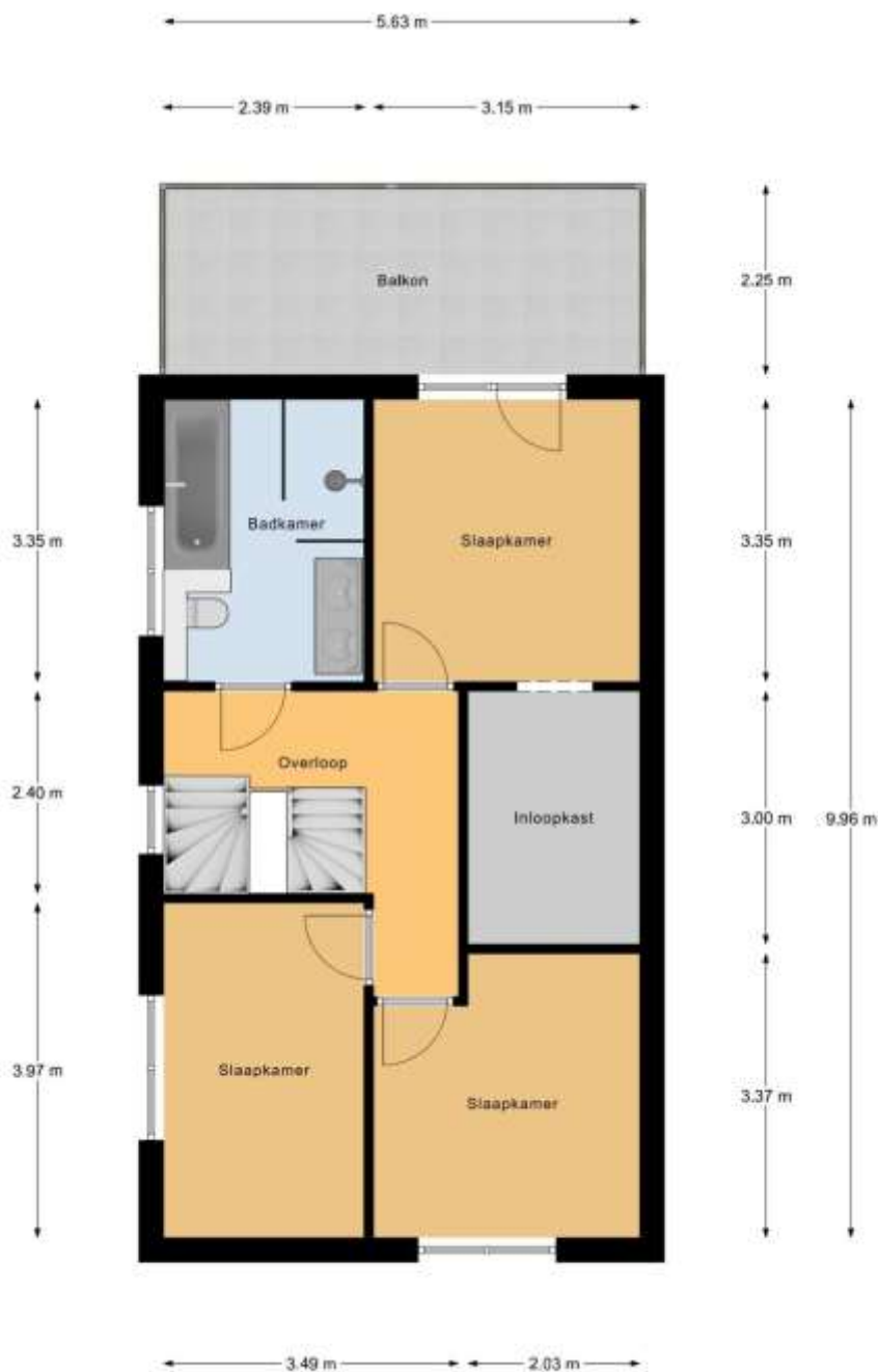
1e Verdieping
