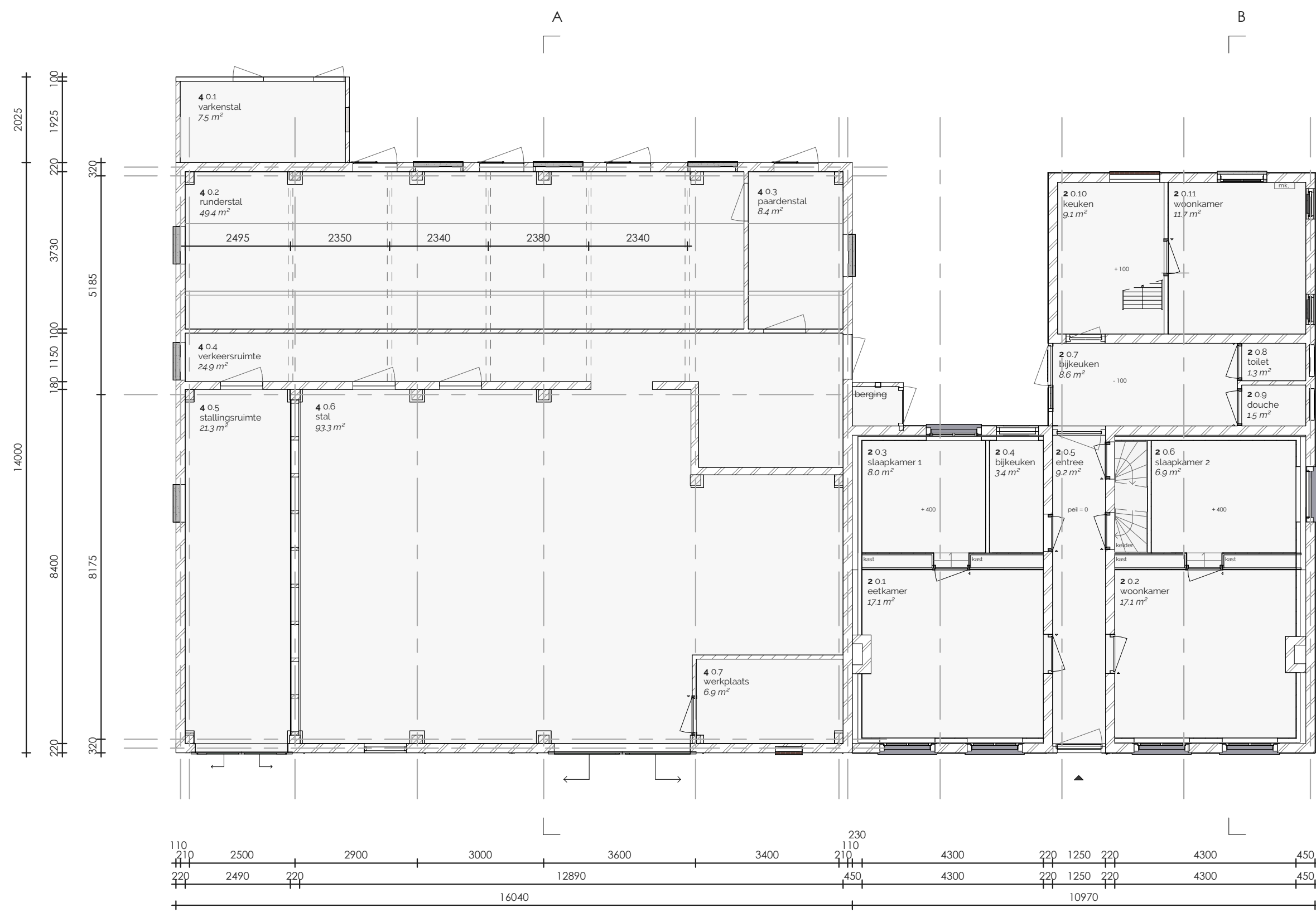
begane grond 1:100
