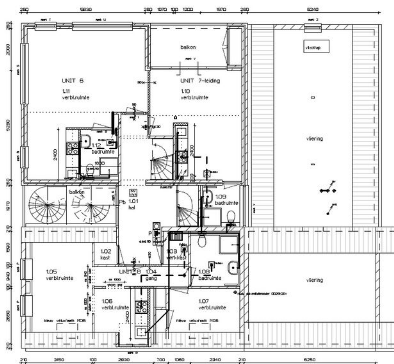
EERSTE VERDIEPING
