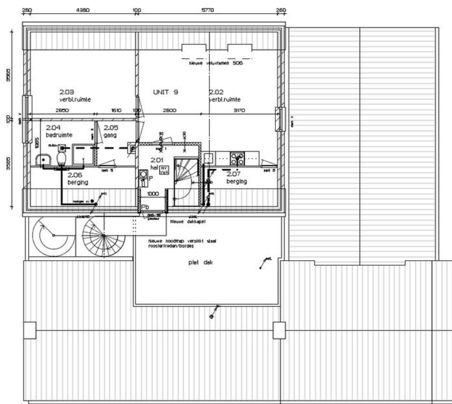
TWEEDE VERDIEPING
