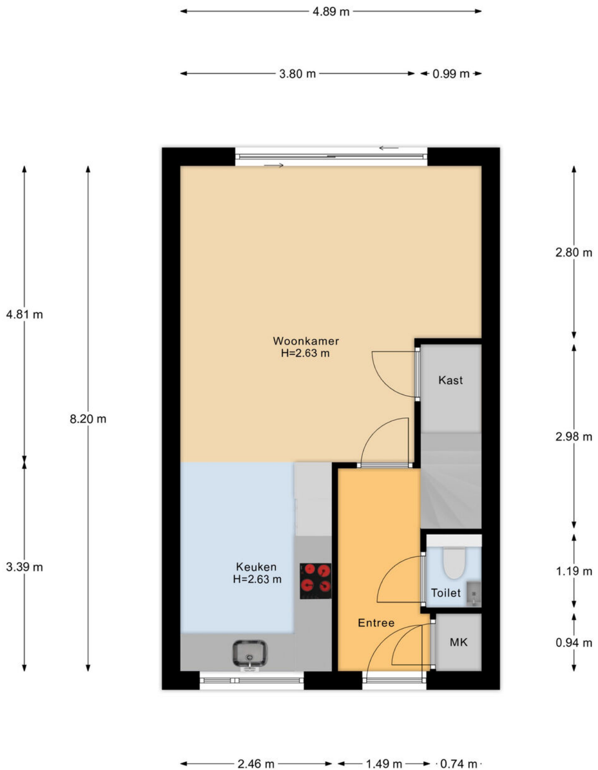
Begane Grond
