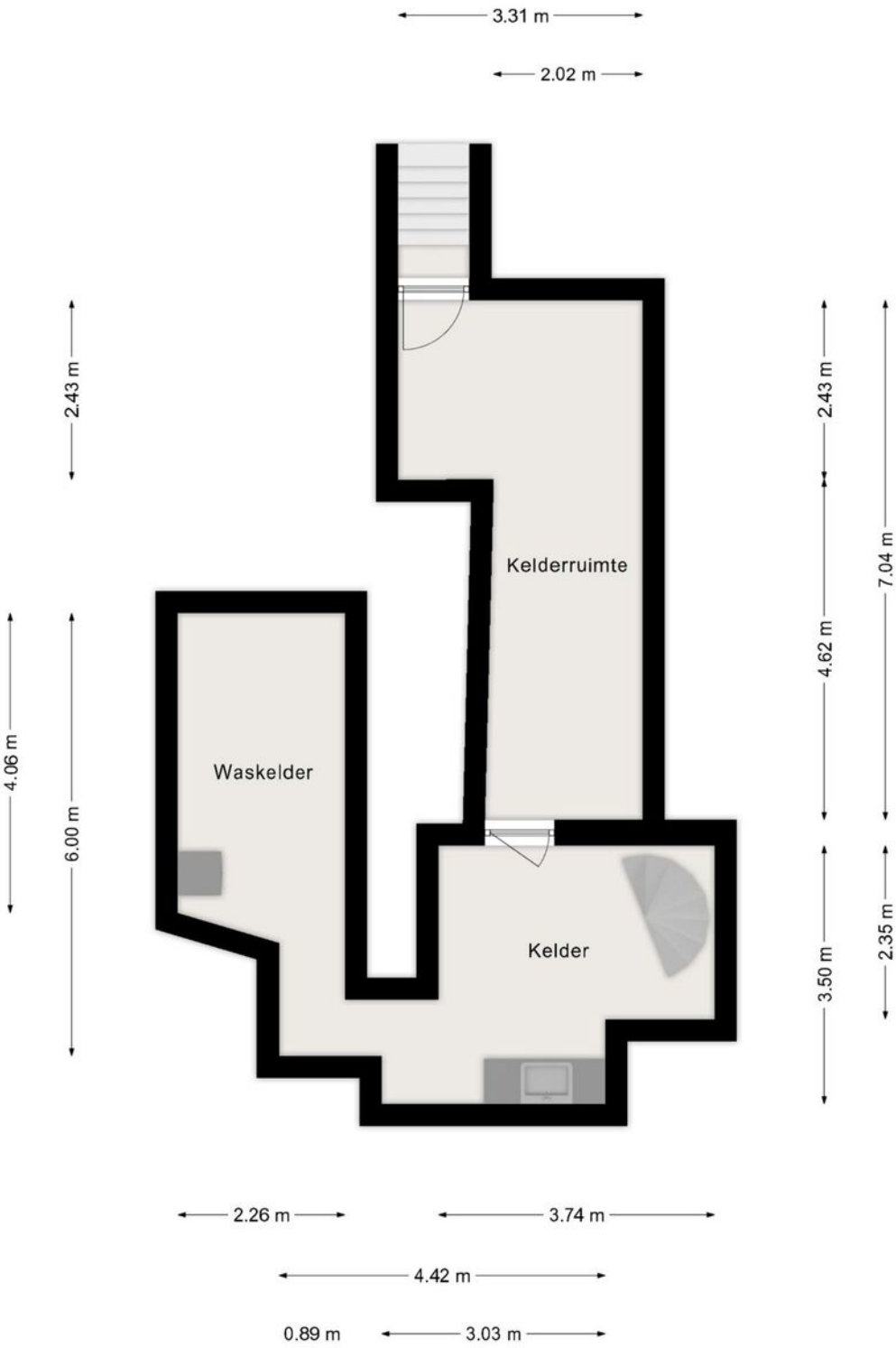
Deze plattegrond dient slechts ter illustratie van de bestaande toestand van de woning. Hier kunnen geen rechten aan worden ontleend.
