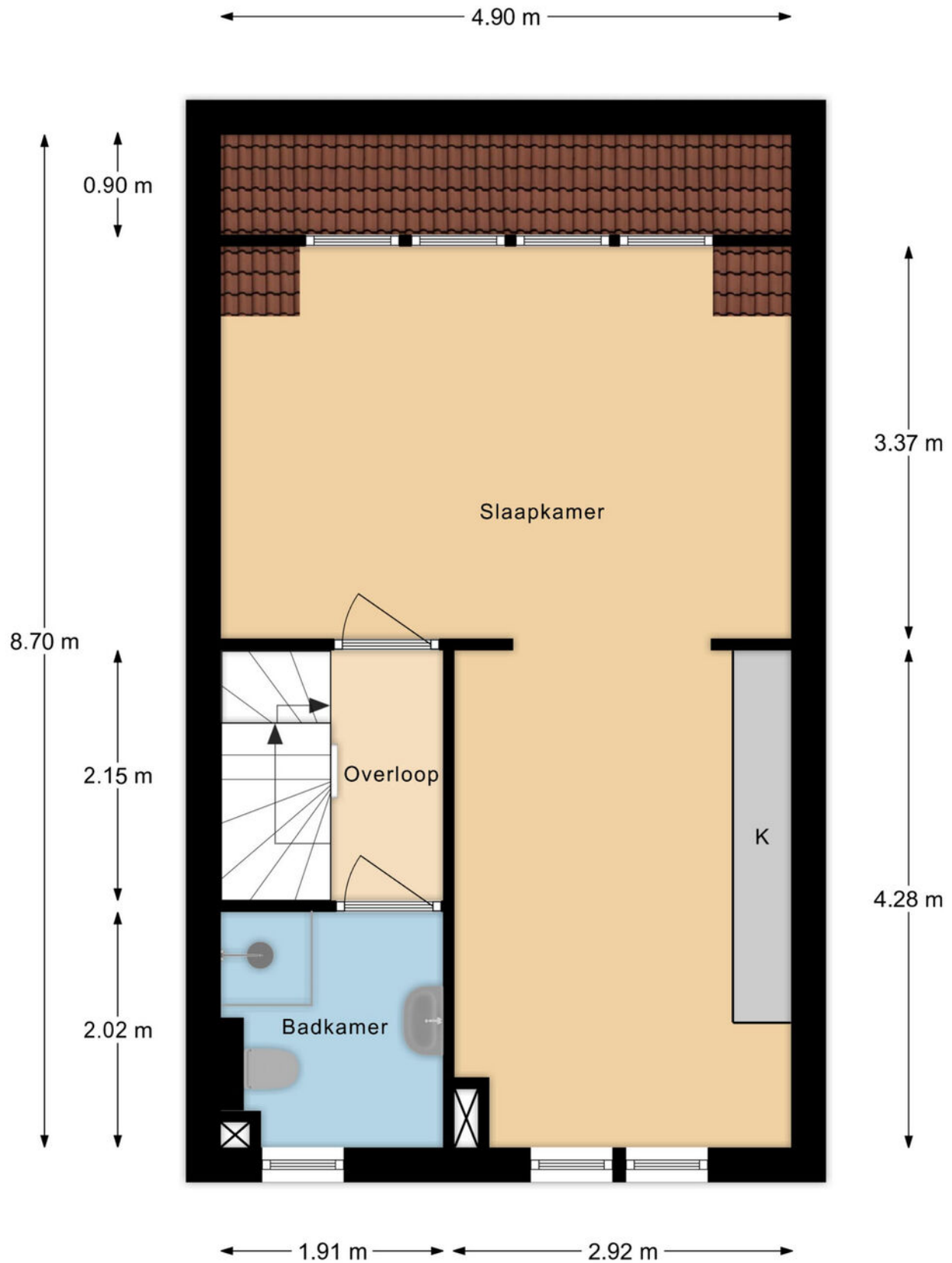
1e Verdieping
