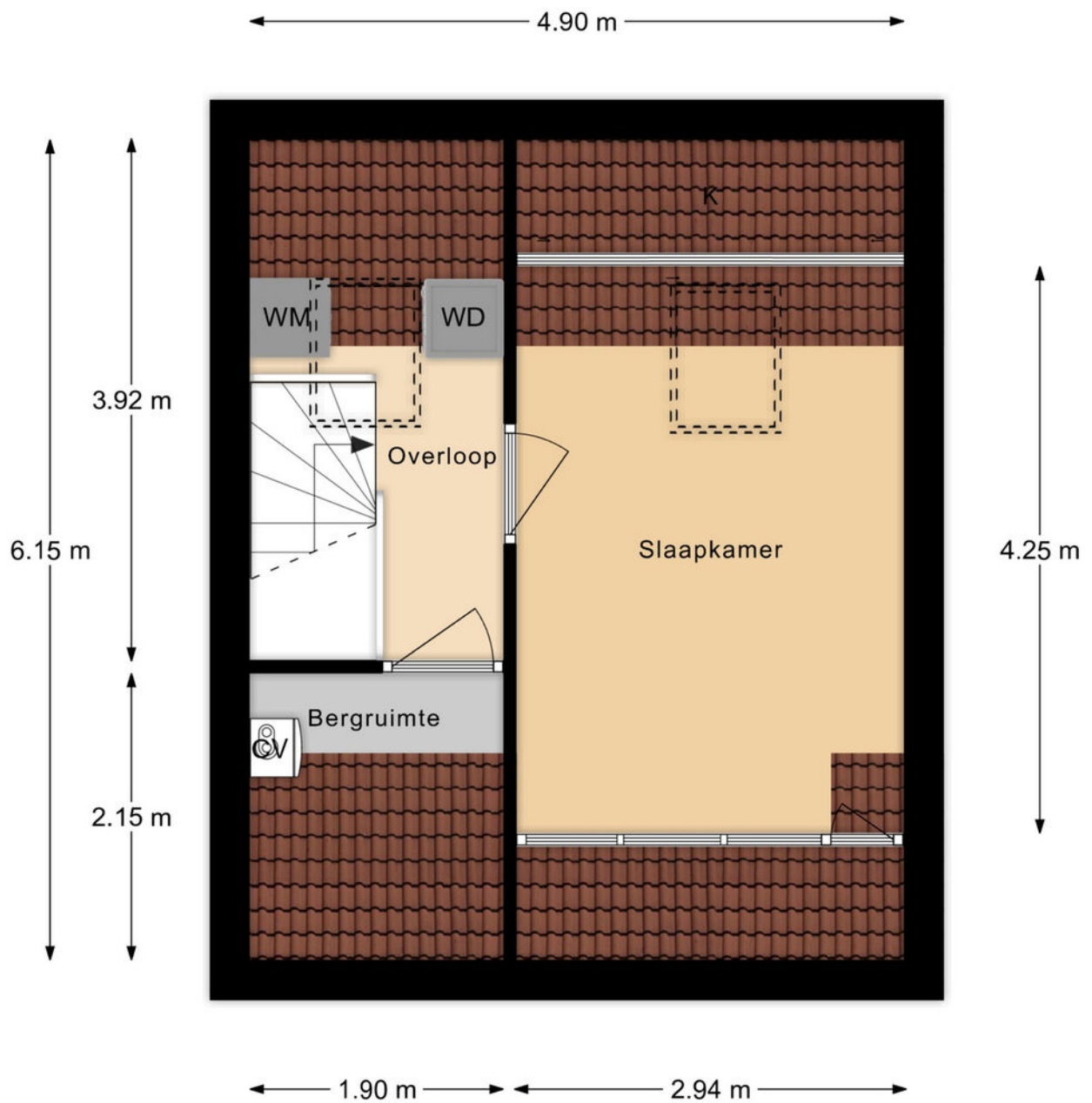
2e Verdieping
