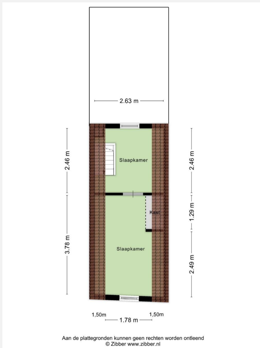
De plattegrond verdieping van de zomerwoning met ca. maatvoeringen.
