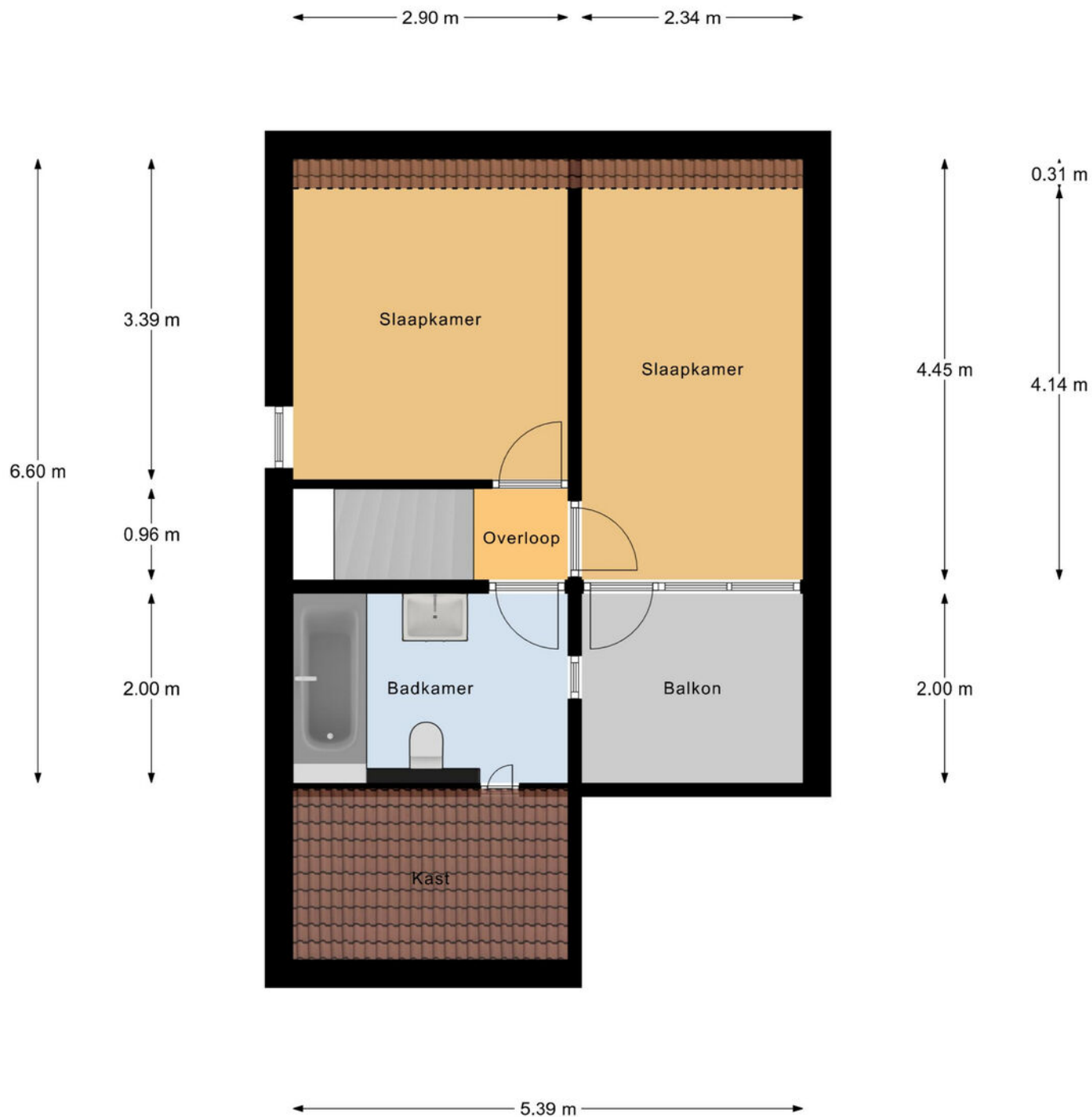
1e Verdieping
