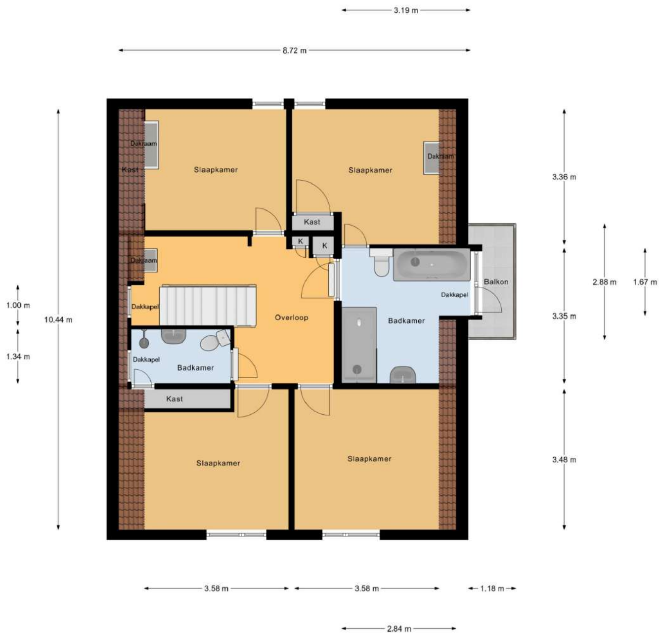
1e Verdieping
