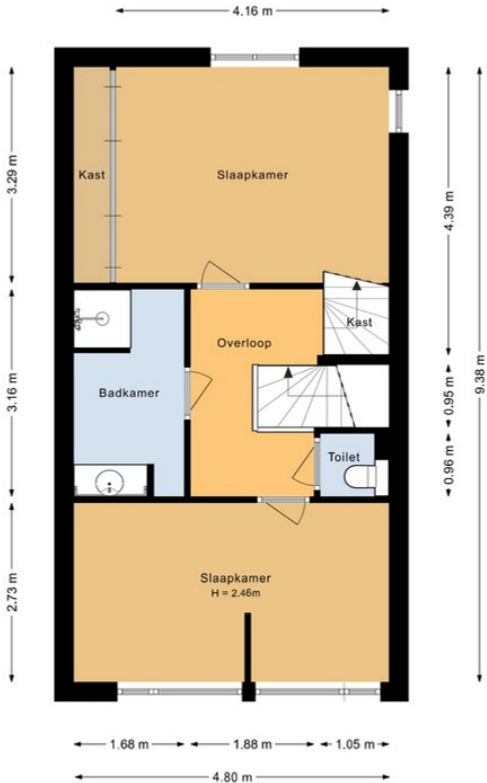
Madura 26 Purmerend Eerste verdieping
