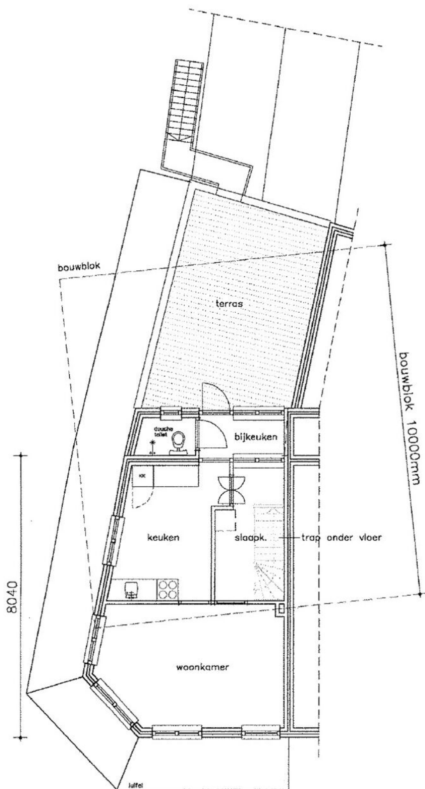
1e verdieping
