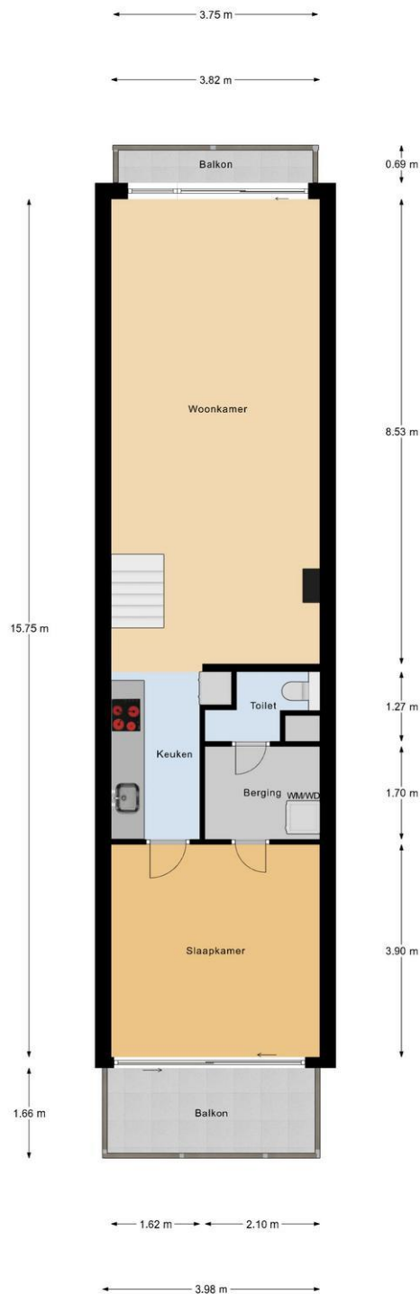
1e Verdieping
