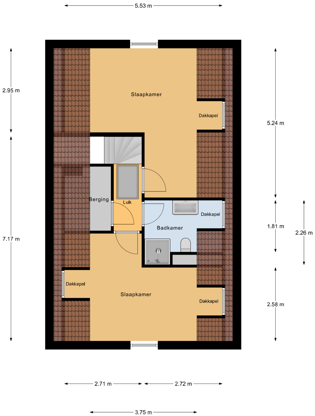
1e Verdieping
