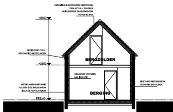
DOORSNEDE B-B
