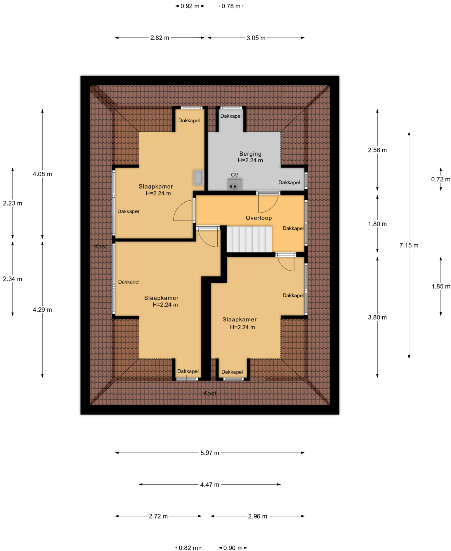
2e Verdieping
