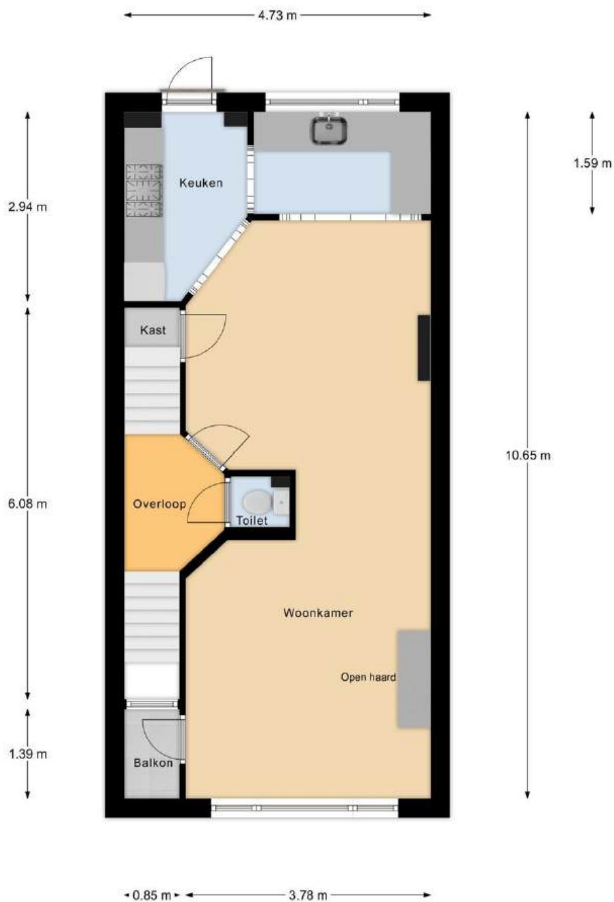
1e Verdieping
