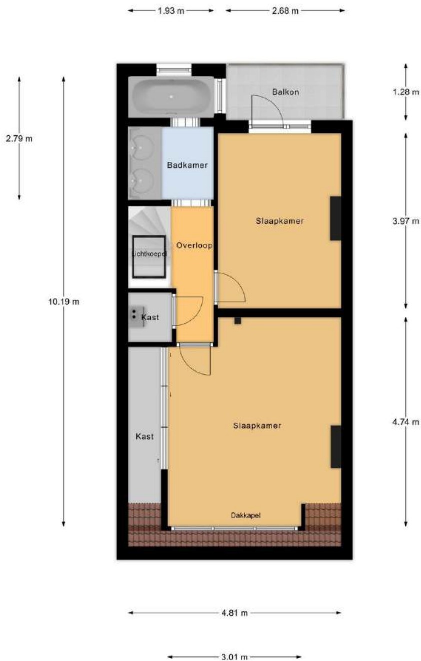
2e Verdieping
