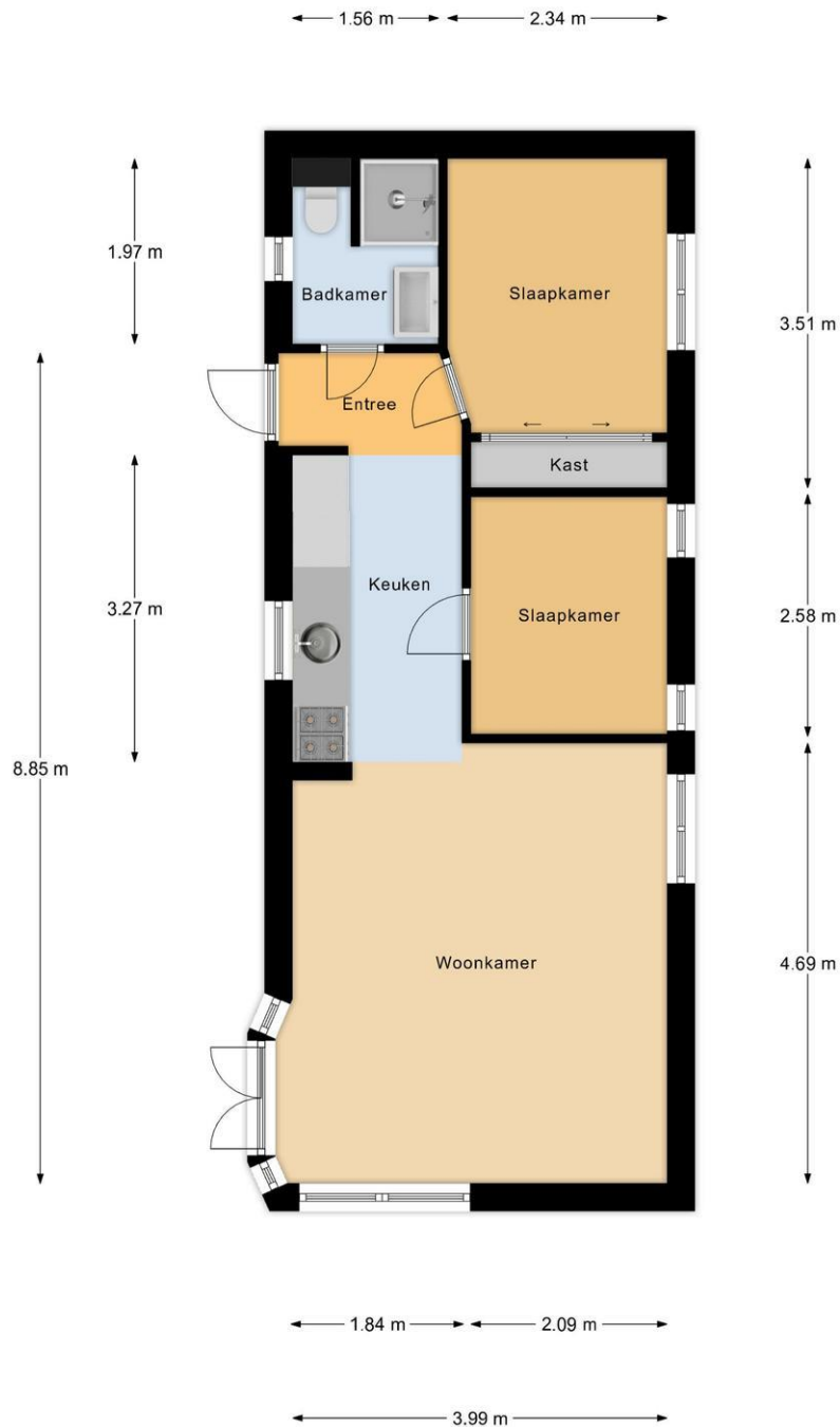
Begane Grond
