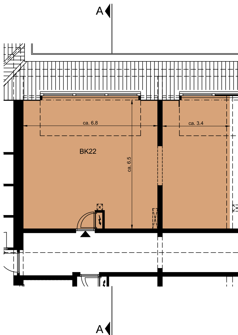
Begane grond
