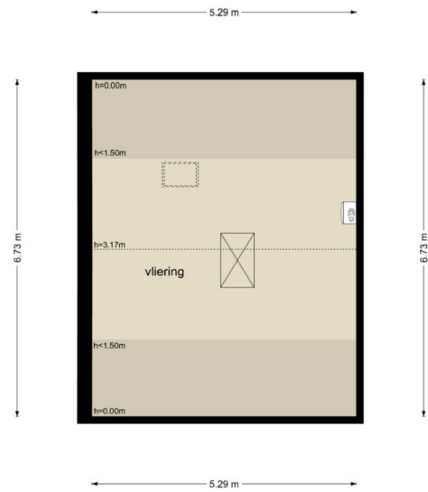
Vliering
