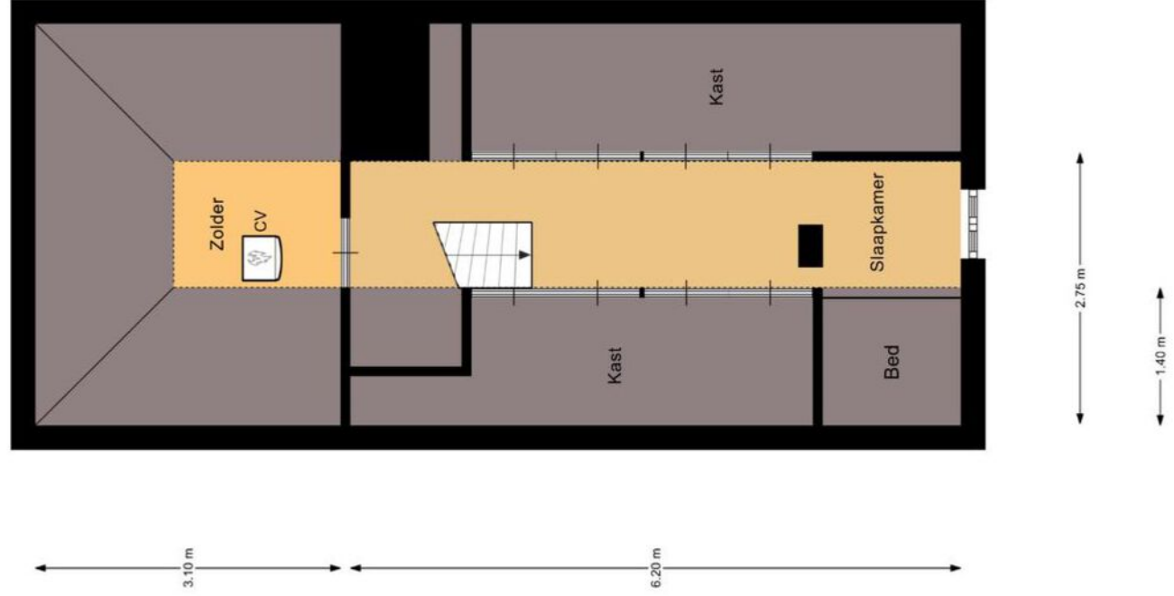
Tweede Verdieping
