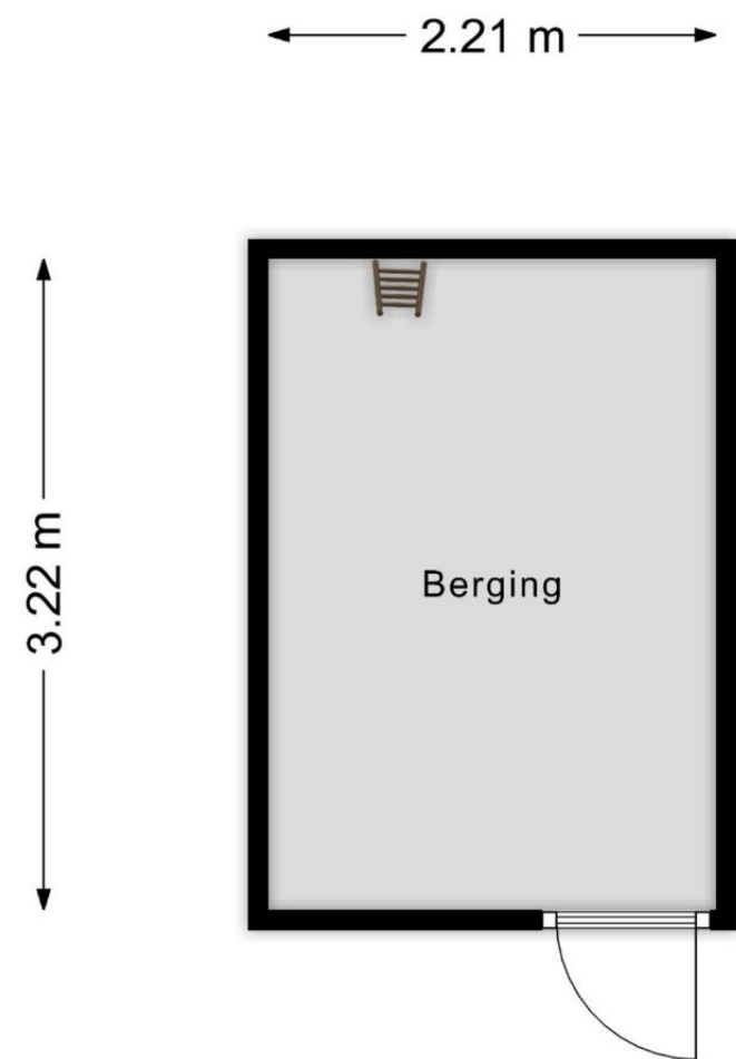
Plattegrond berging Aan deze tekening kunnen geen rechten worden ontleend
