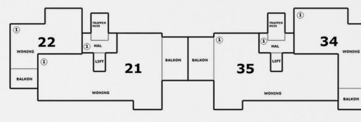
3e verdieping
