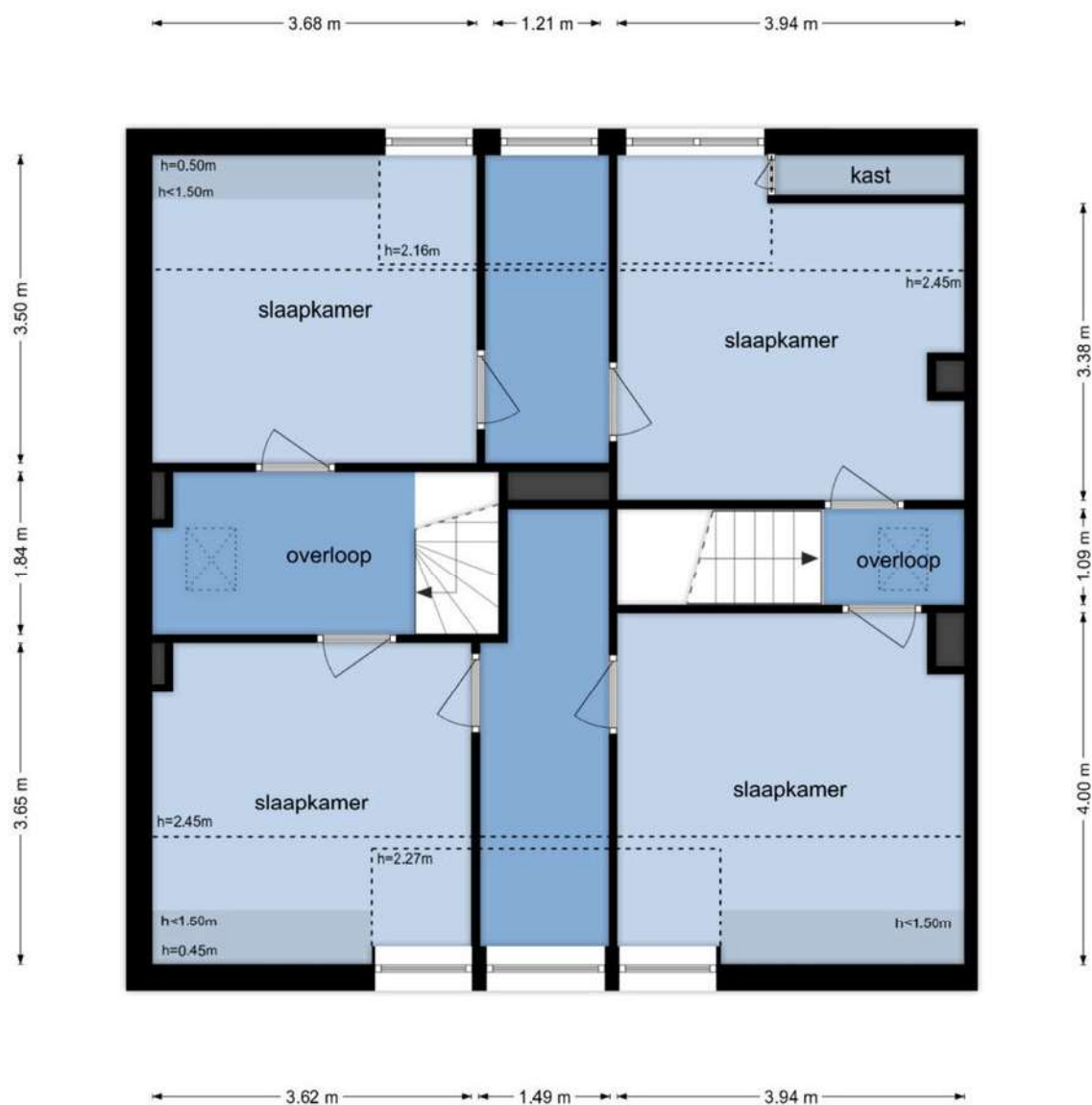
Stokkumseweg 10 - 's Heerenberg Eerste Verdieping
