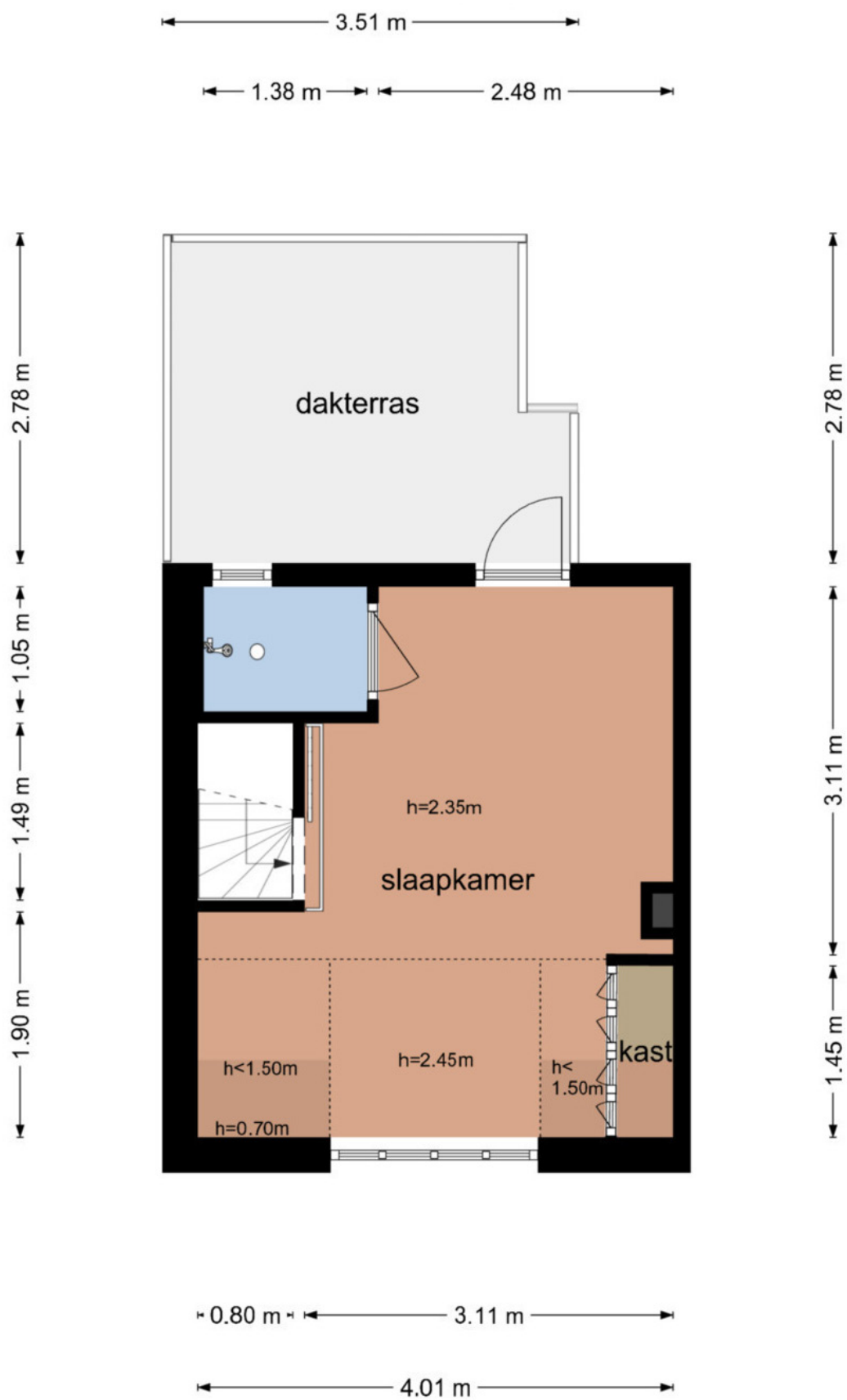
Eerste verdieping
