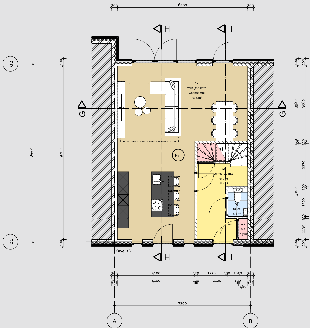
- BEGANE GROND -
