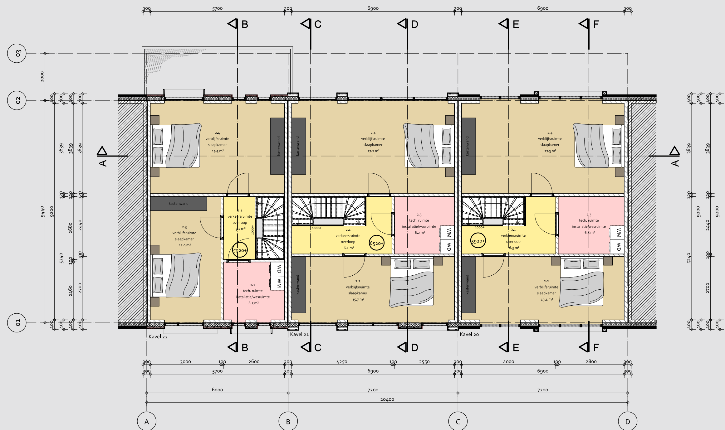
- 2e VERDIEPING -
