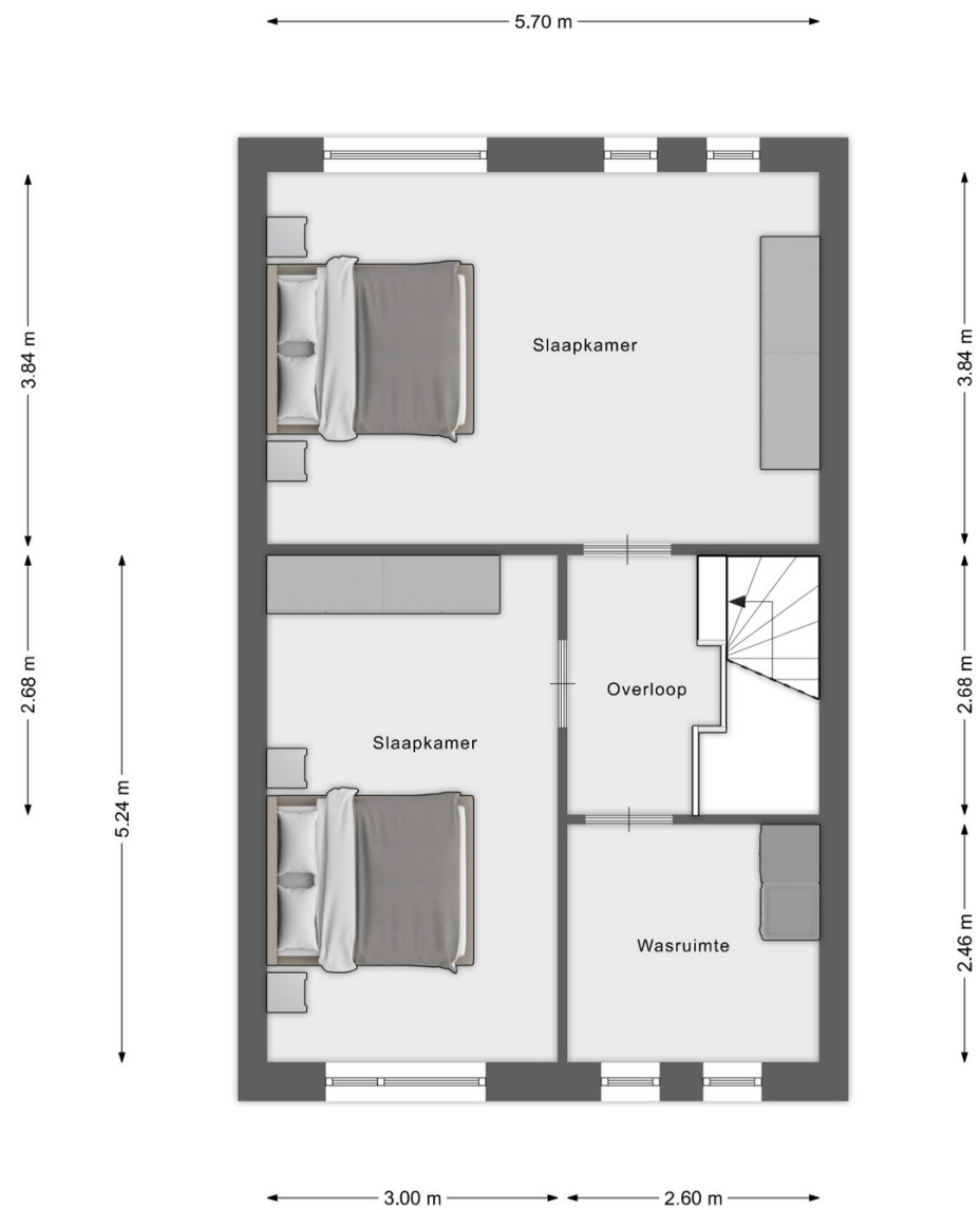
2E VERDIEPING
