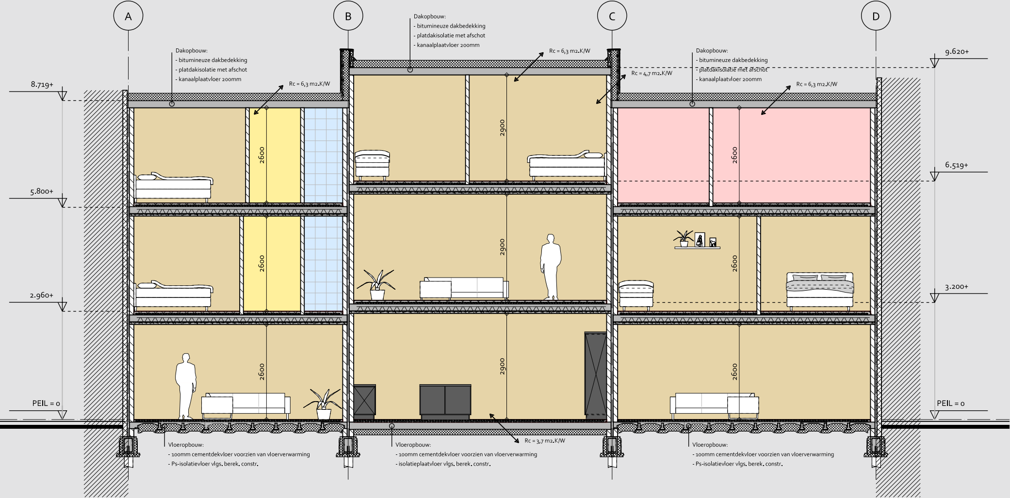
- DOORSNEDE A-A -
