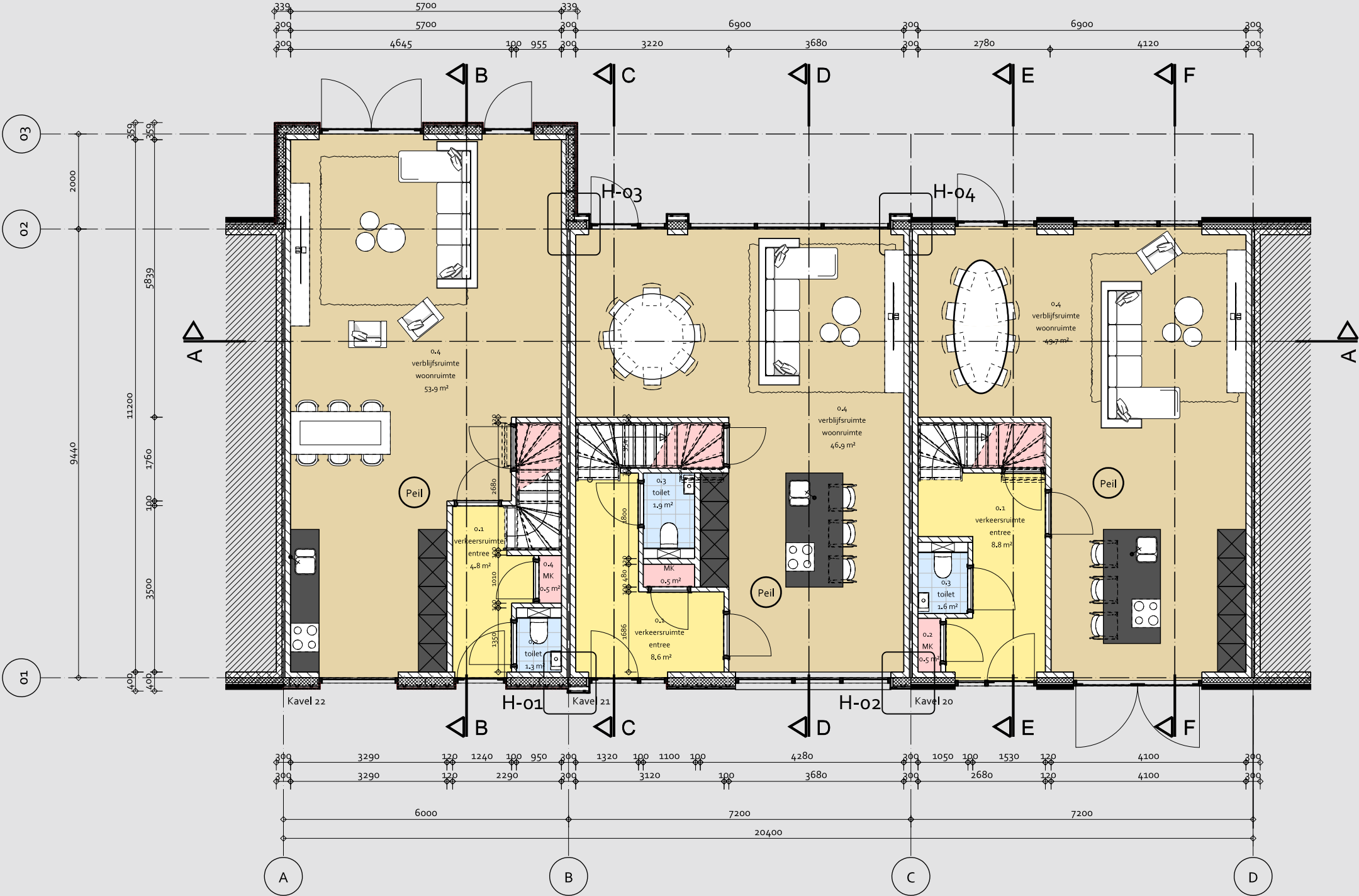
- BEGANE GROND -
