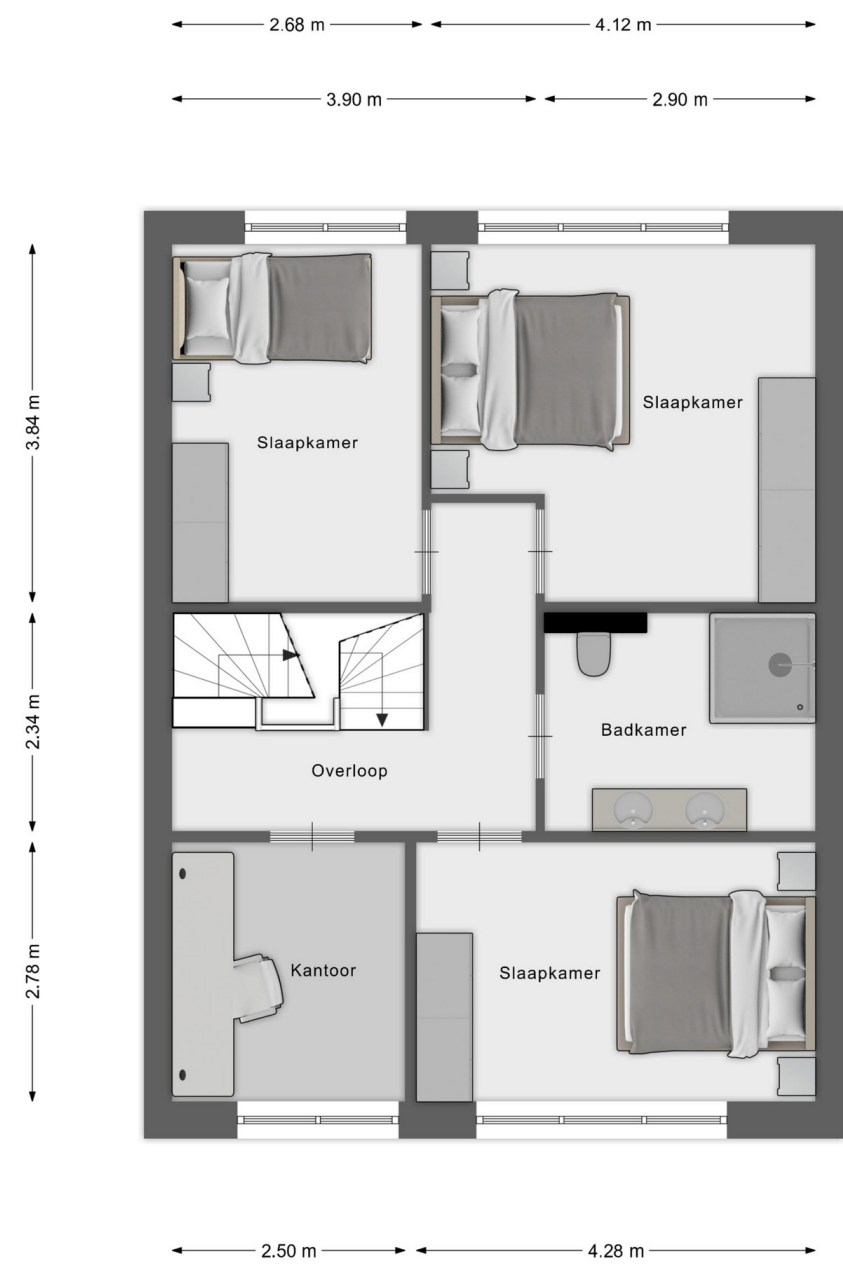
1E VERDIEPING
