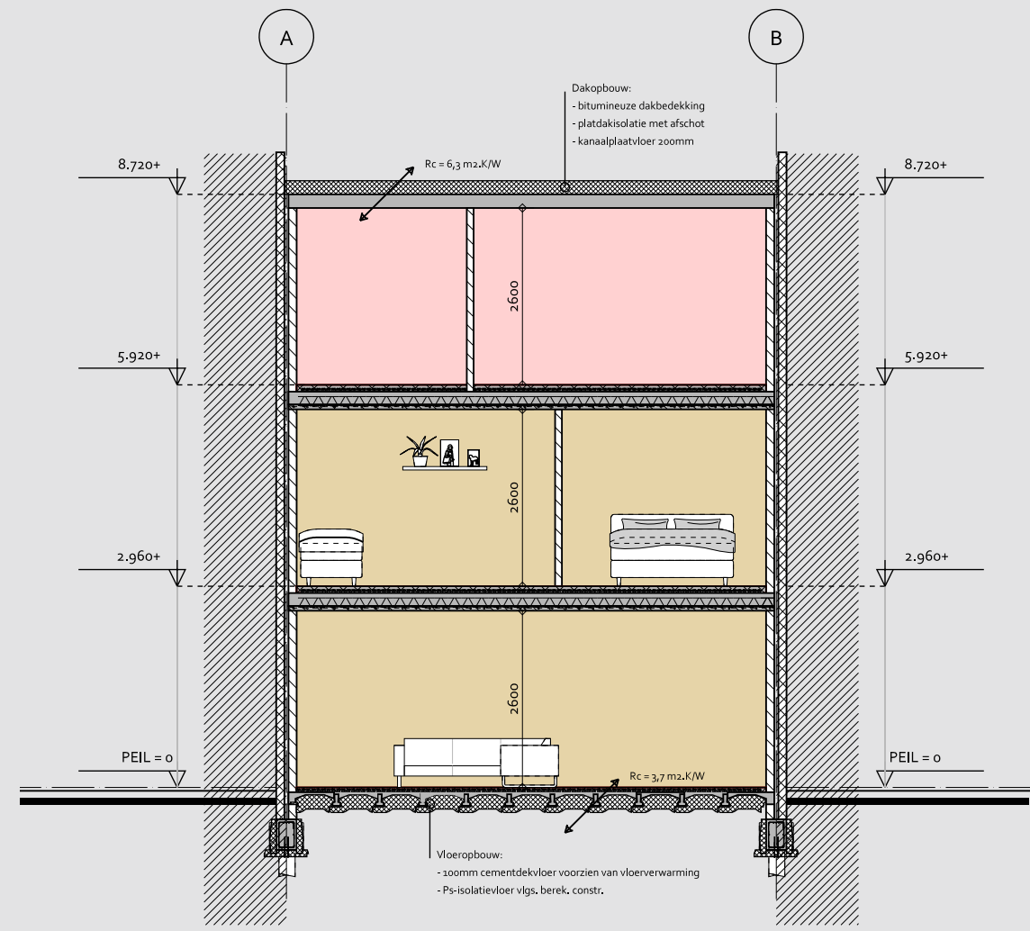
- DOORSNEDE G-G - - KAVEL 26 -
