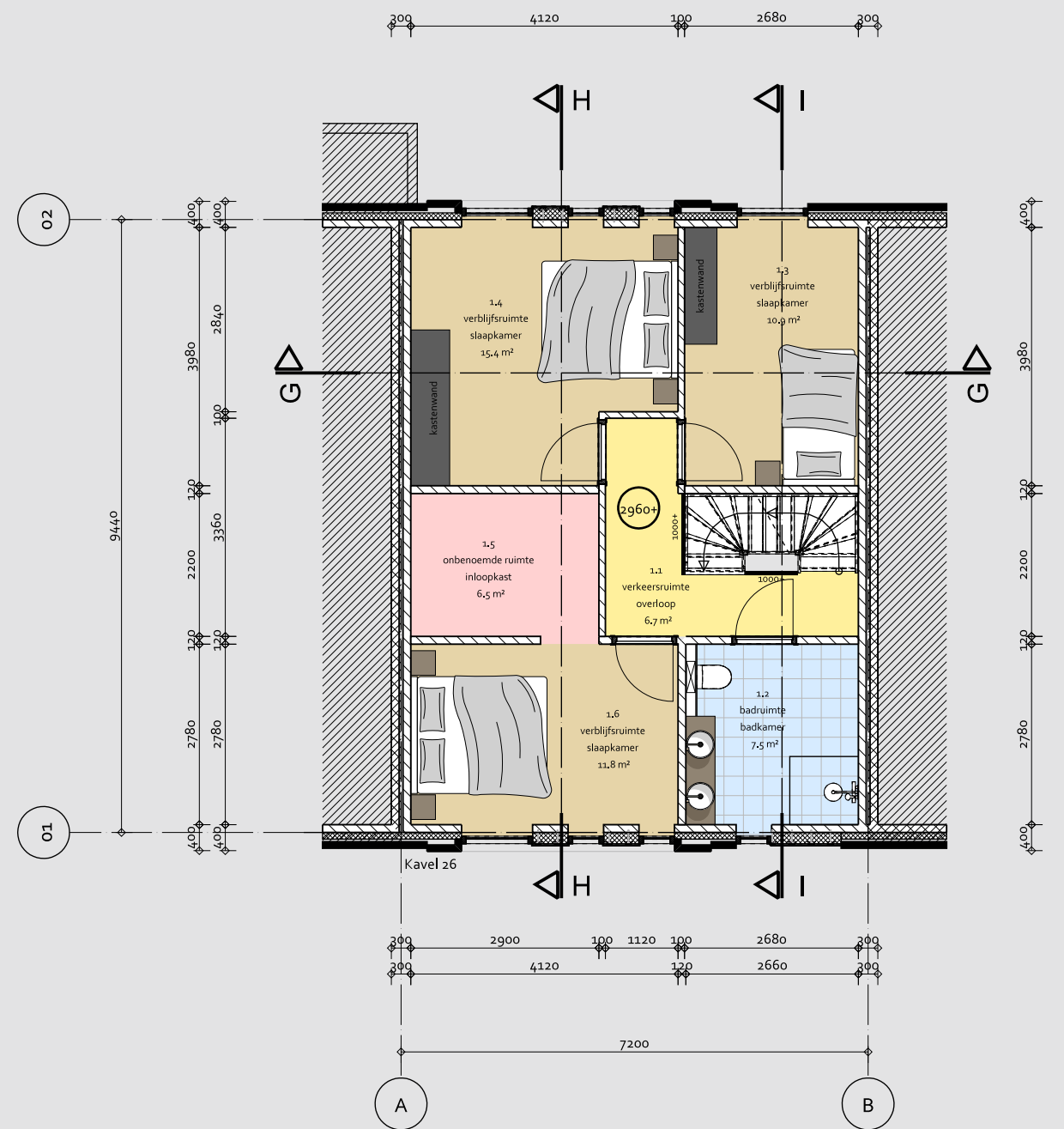
1e VERDIEPING -
