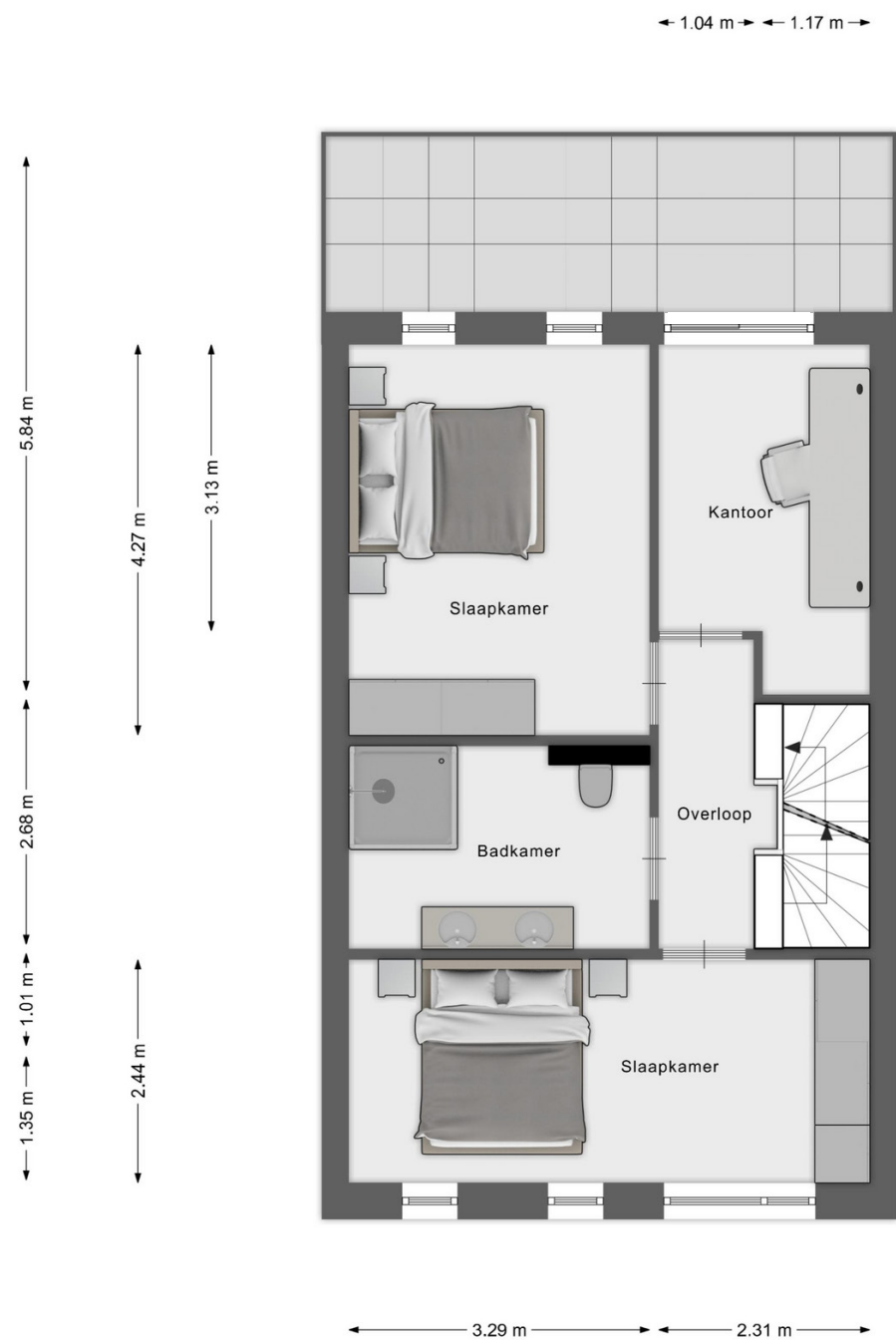
1E VERDIEPING
