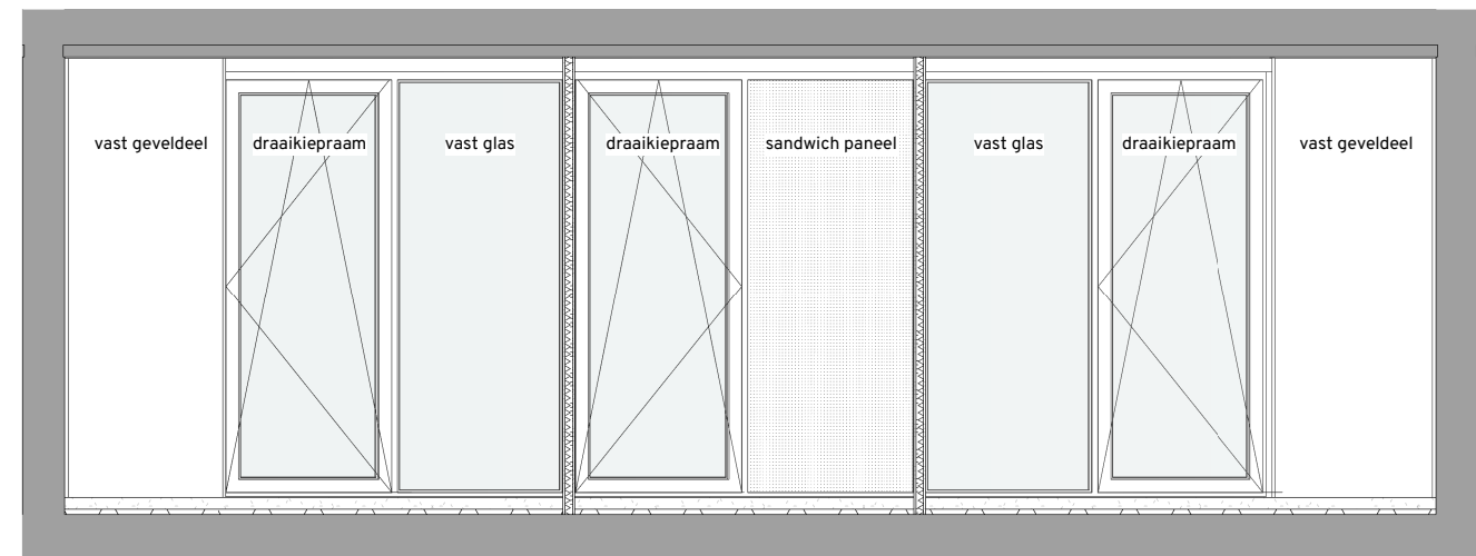
doorsnede bouwnummer 207, 307
