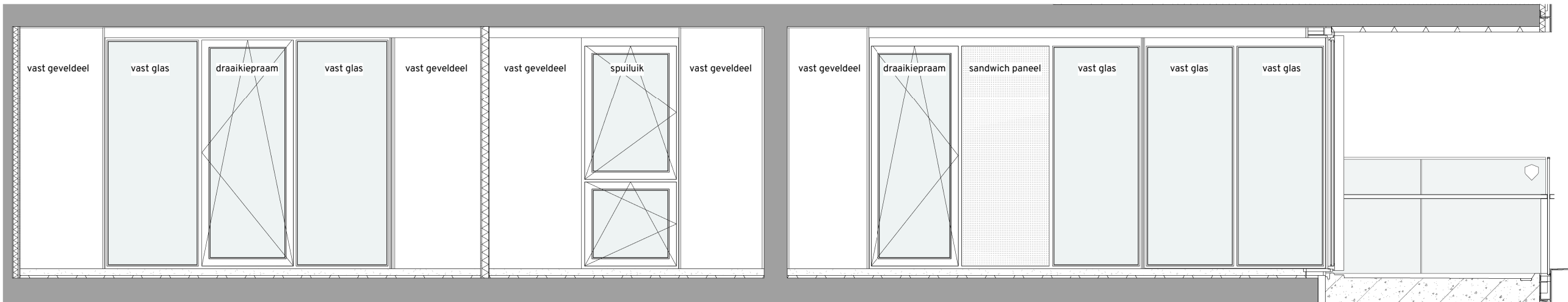
doorsnede BB bouwnummer 703
