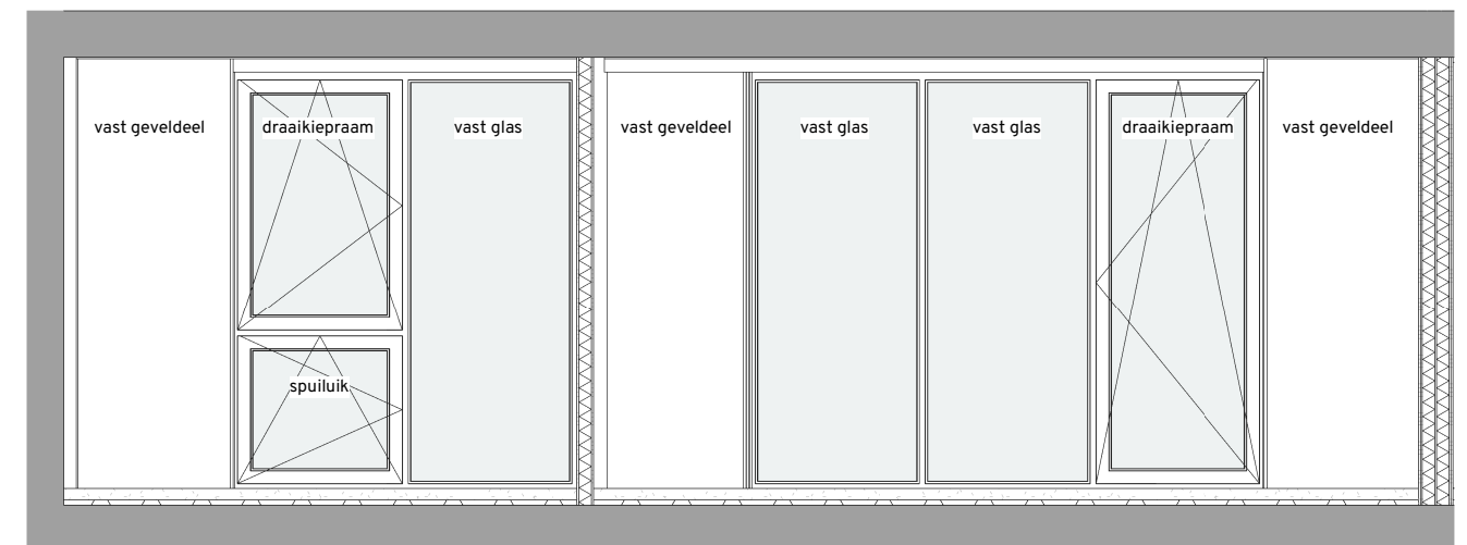
doorsnede bouwnummer 505
