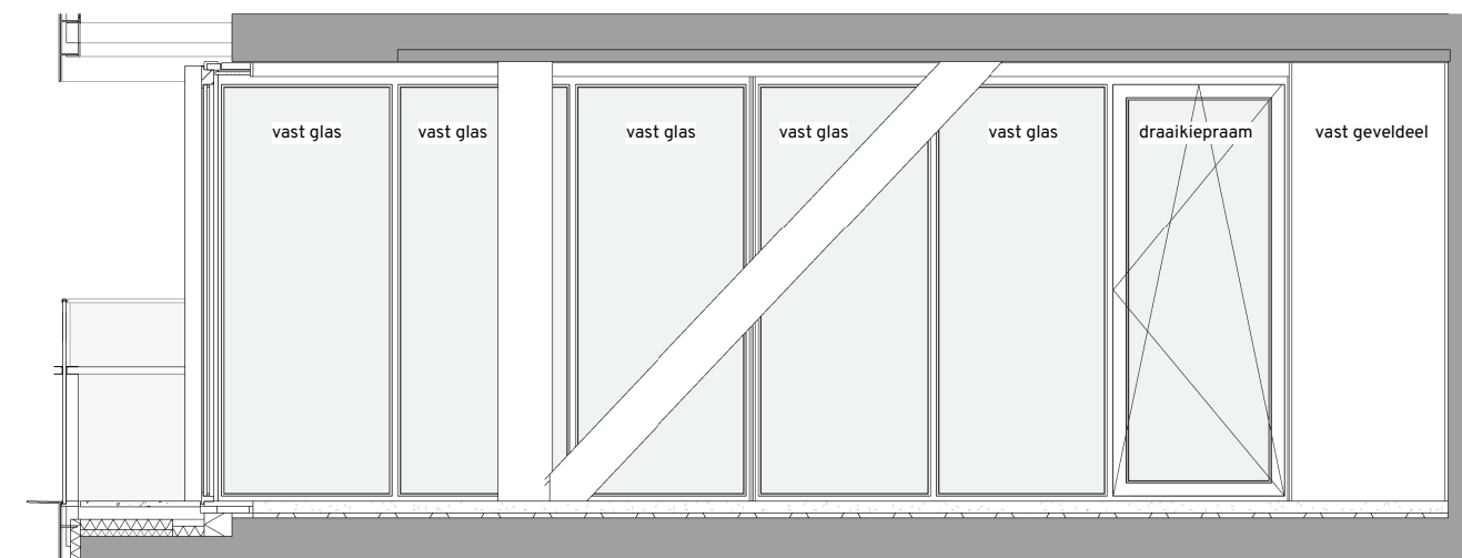
doorsnede bouwnummer 204
