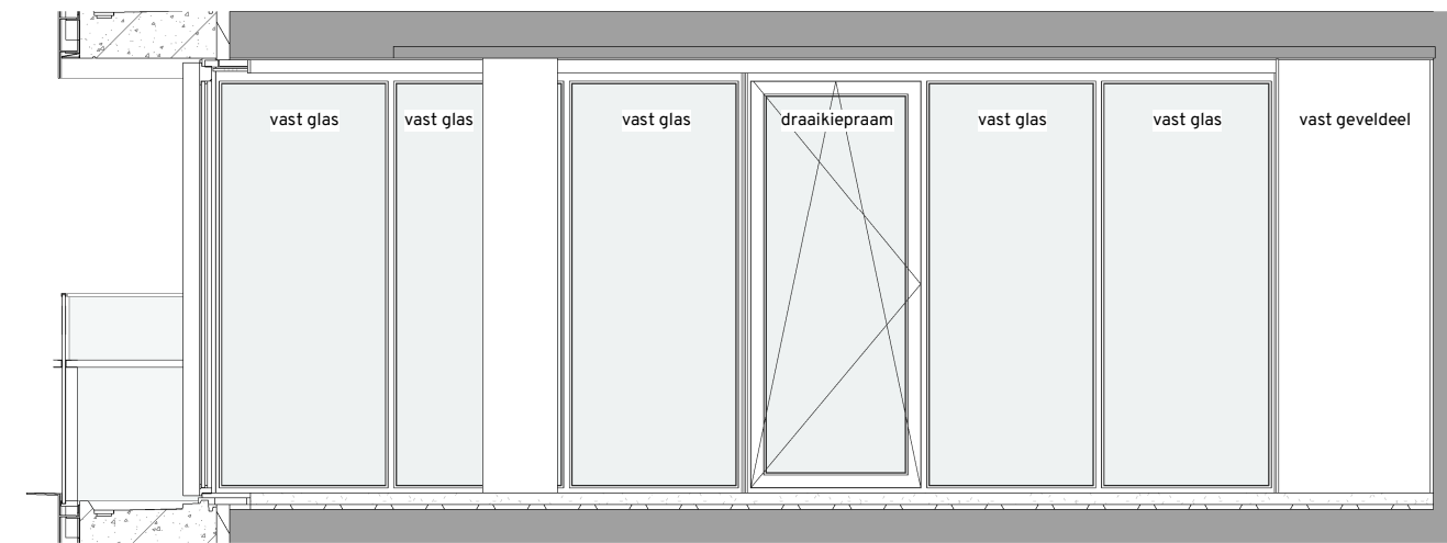
doorsnede bouwnummer 404
