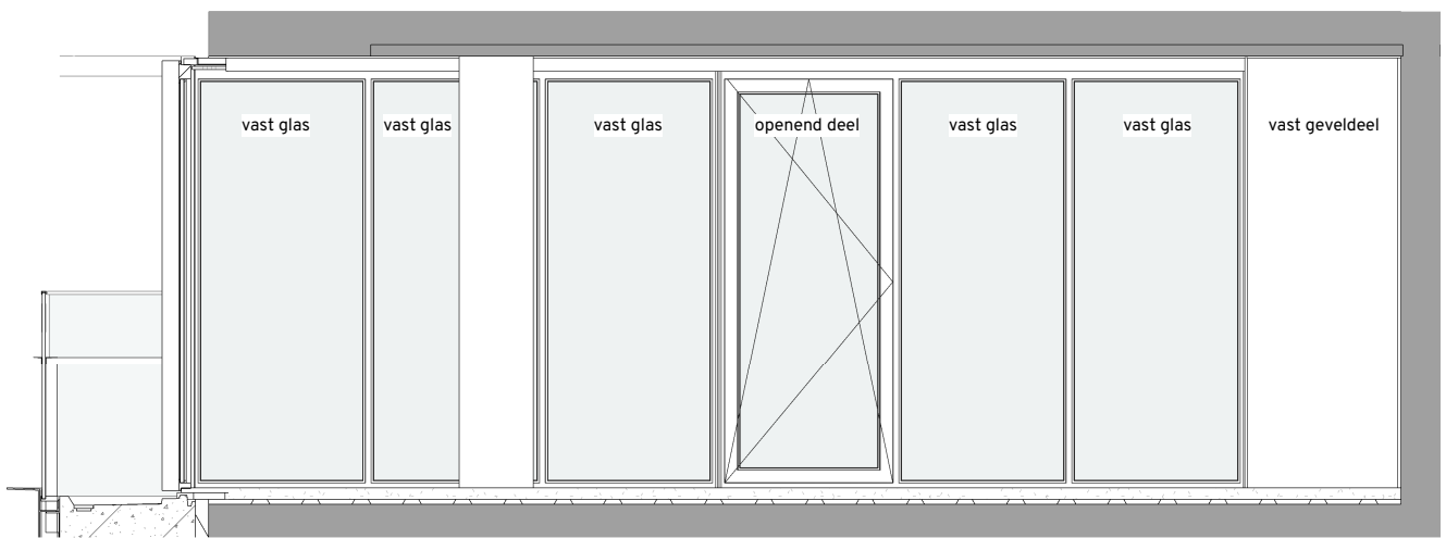
doorsnede AA bouwnummer 504
