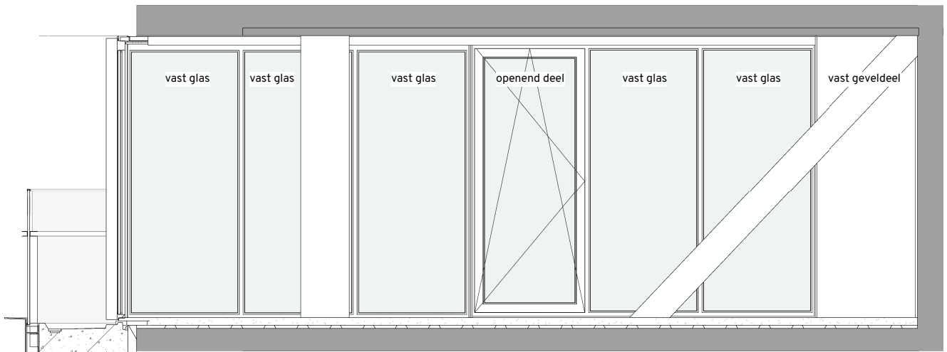
doorsnede AA bouwnummer 304
