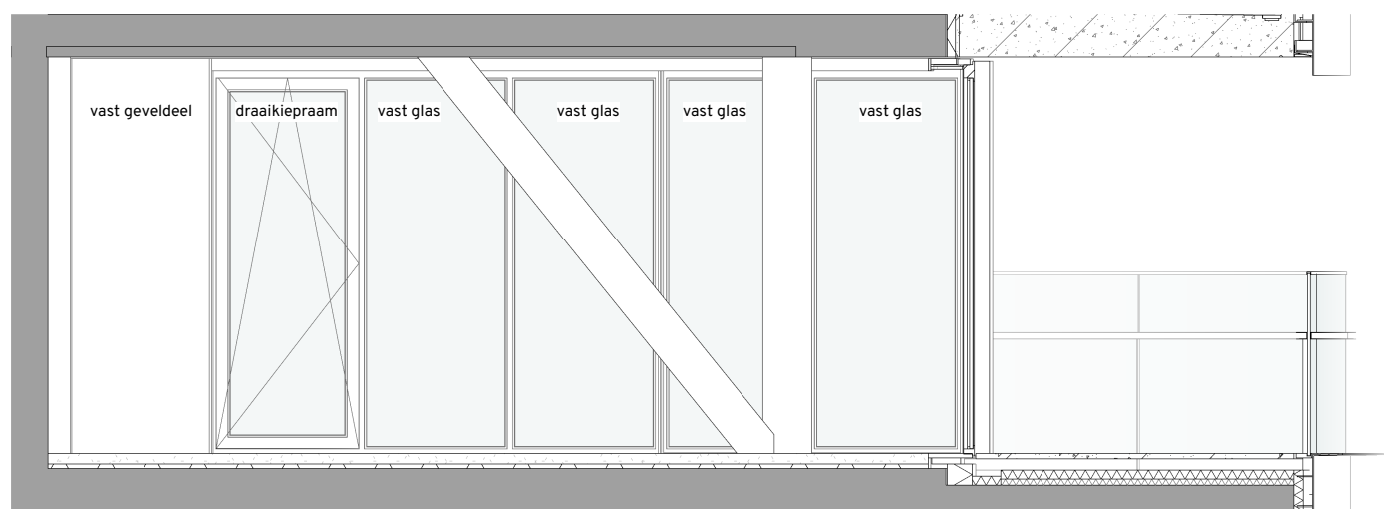
doorsnede bouwnummer 203
