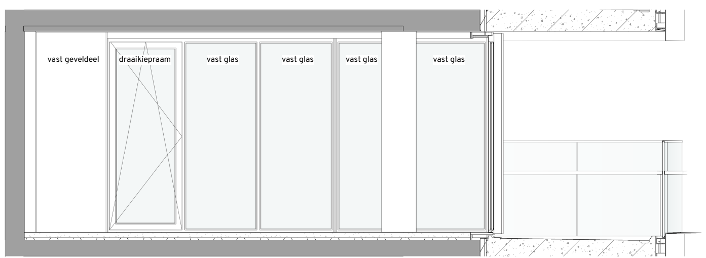
doorsnede bouwnummer 403
