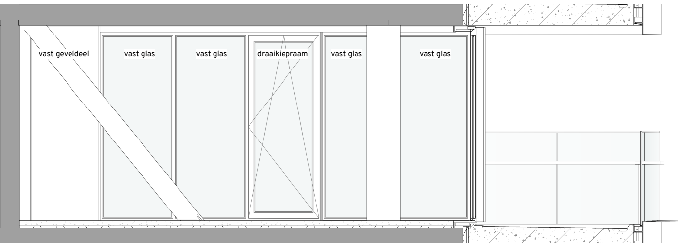
doorsnede bouwnummer 303
