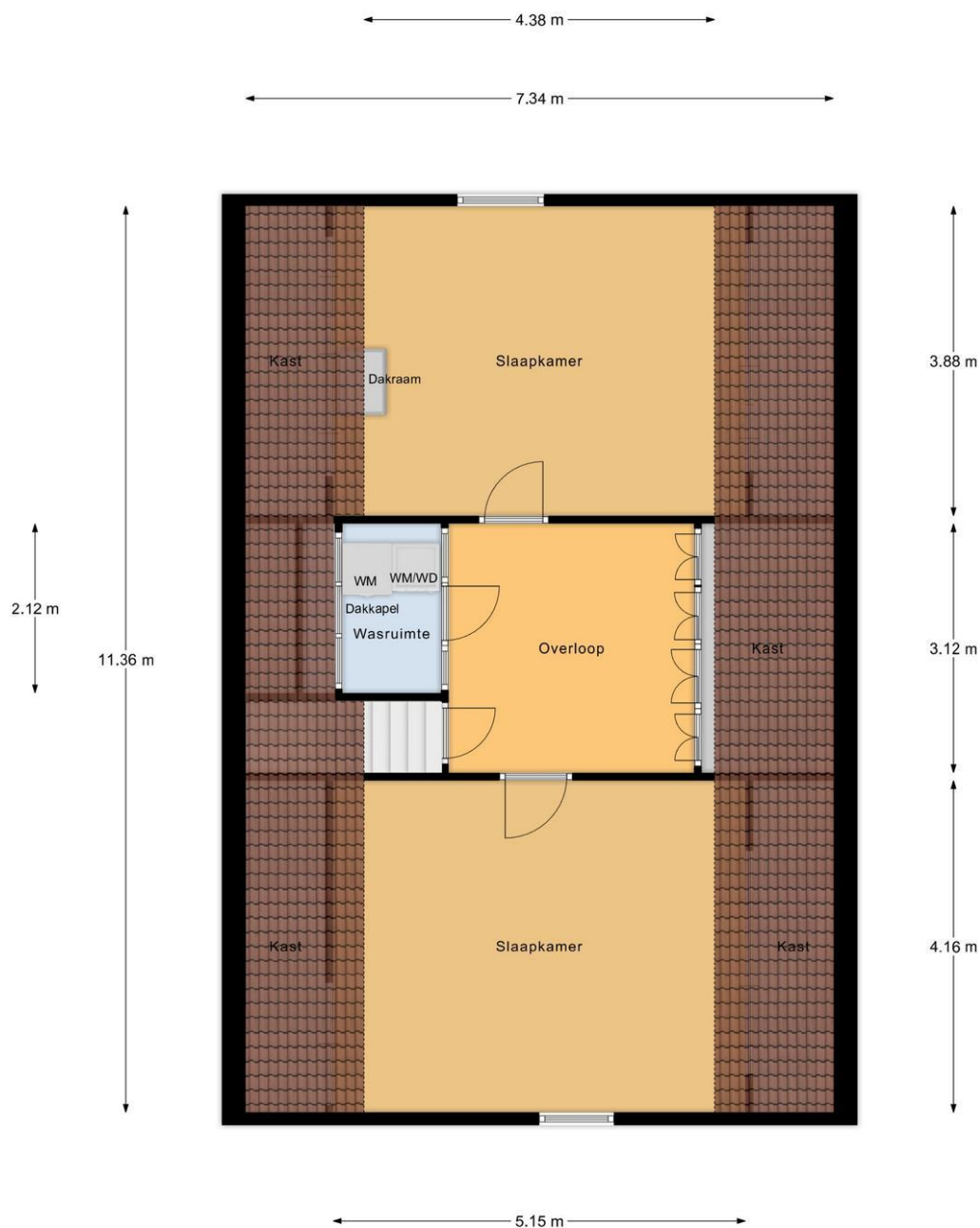
1e Verdieping
