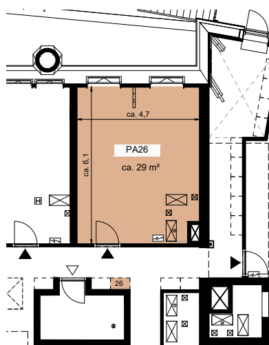
Tweede verdieping
