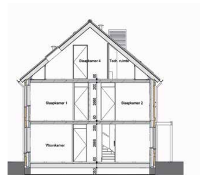
Doorsnede
