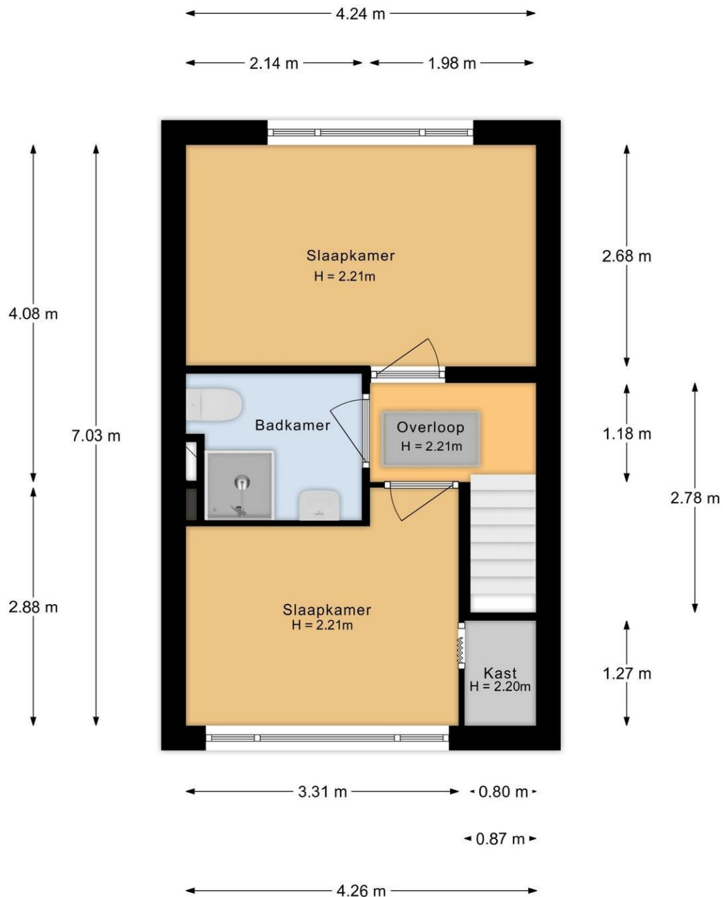
Optie plattegrond badkamer eerste verdieping
