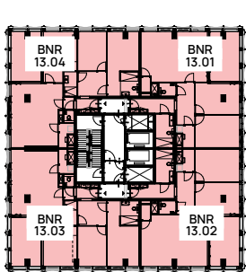
13e verdieping
