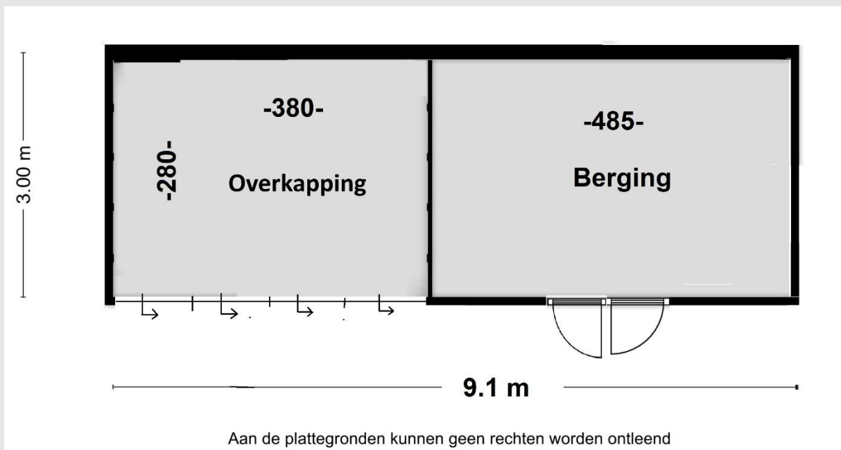
Plattegrond van de overkapping met ca. maatvoering.
