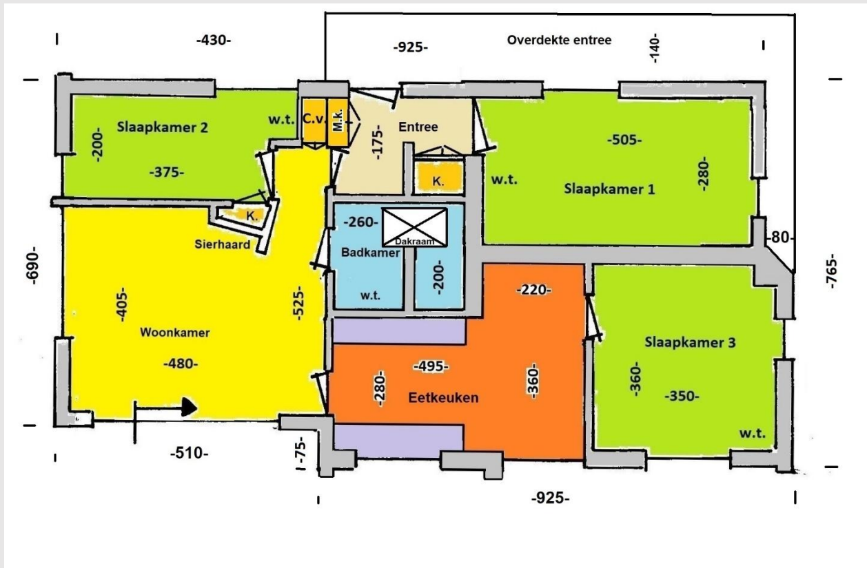
Plattegrond van de woning met ca. maatvoering.
