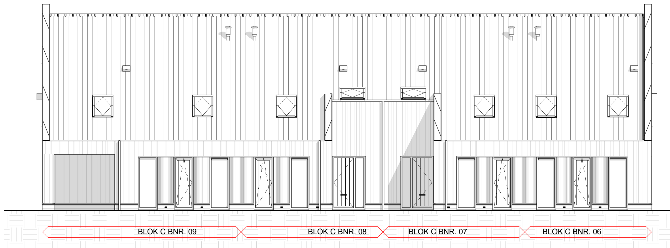
voorgevel
