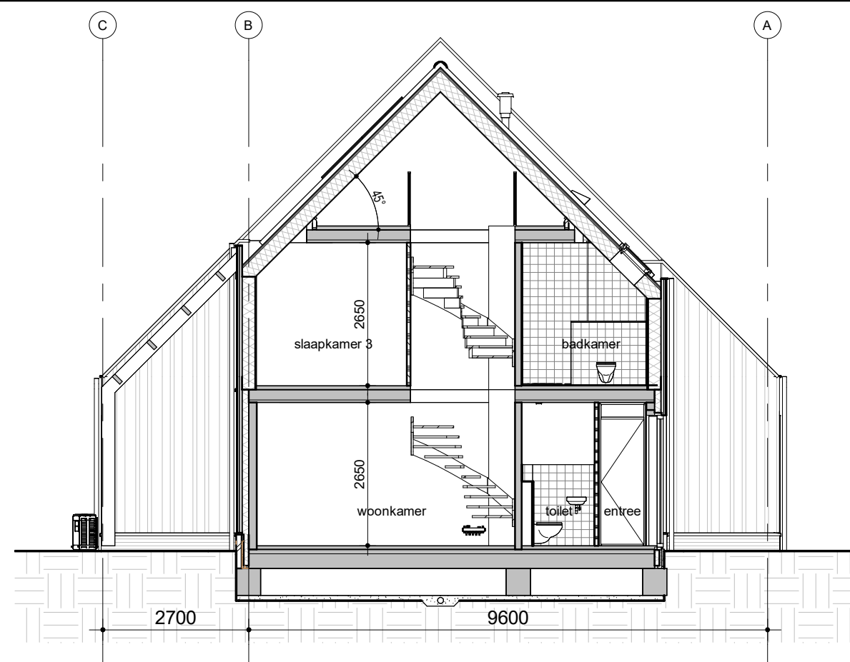
Doorsnede B
