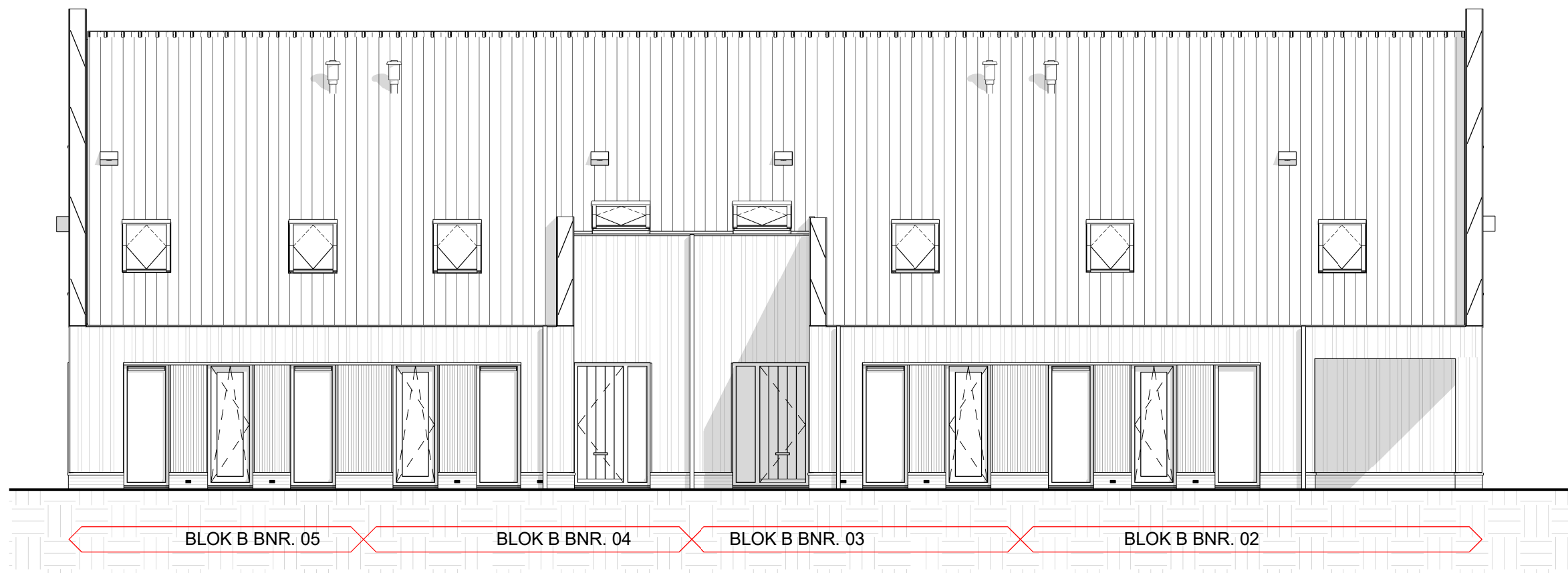
voorgevel
