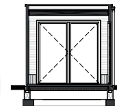
DOORSNEDEN
