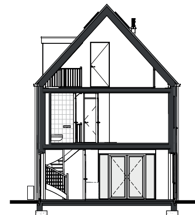
DOORSNEDE
